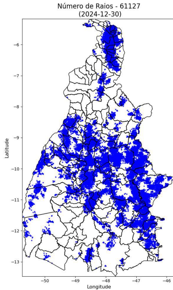
Figura 2 – Mapa de descargas atmosféricas para os dias 08/12 a 30/12.
