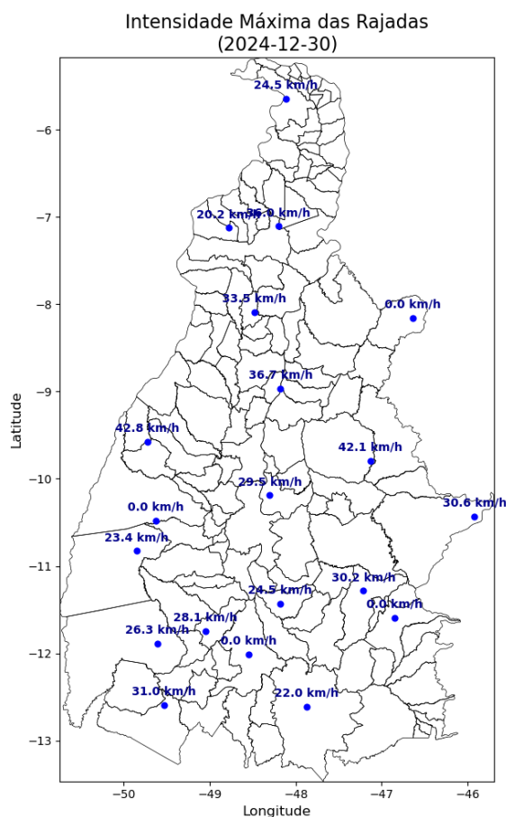
Figura 4 – Mapa da intensidade máxima das rajadas para os dias 08/12 a 30/12.
