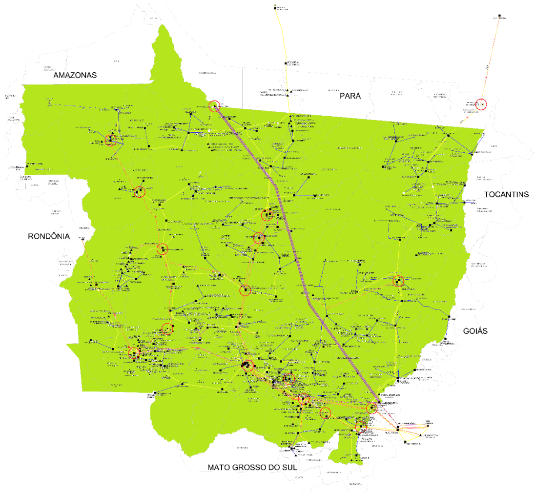
Figura 2 - Diagrama unifilar da subtransmissão com municípios do estado afetados pelos eventos (em verde - todos, conforme Laudos).
