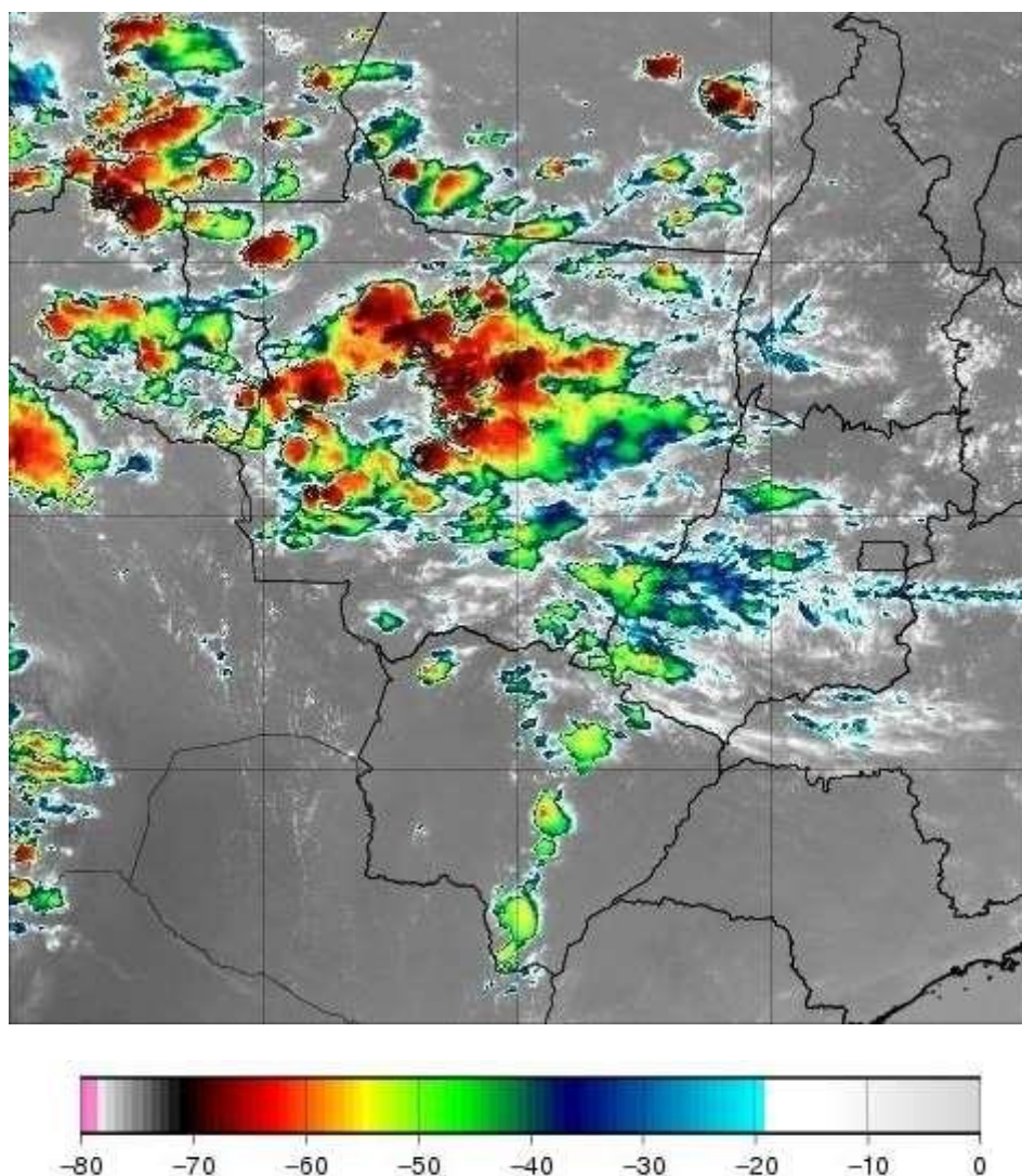
Figura 1 - Imagem de satélite no infravermelho com realce do satélite GOES-16 durante um dos períodos de máxima intensidade do evento às 20:00 UT do dia 22/09. As cores indicam diferentes temperaturas dos topos das nuvens.
