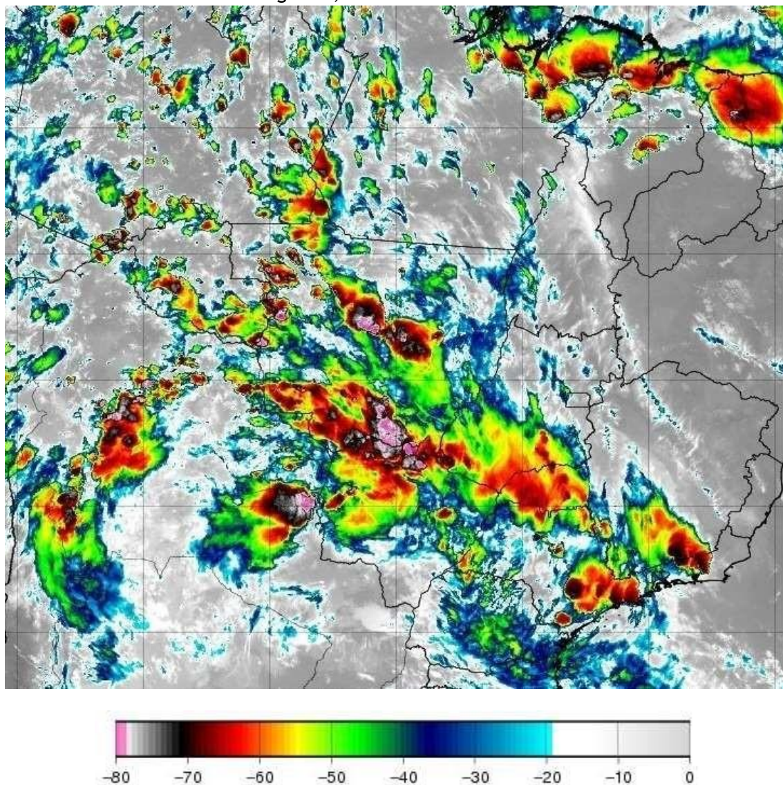
Figura 1 - Imagem de satélite no infravermelho com realce do satélite GOES-16 durante um dos períodos de máxima intensidade do evento às 22:00 UT do dia 12/02. As cores indicam diferentes temperaturas dos topos das nuvens.
