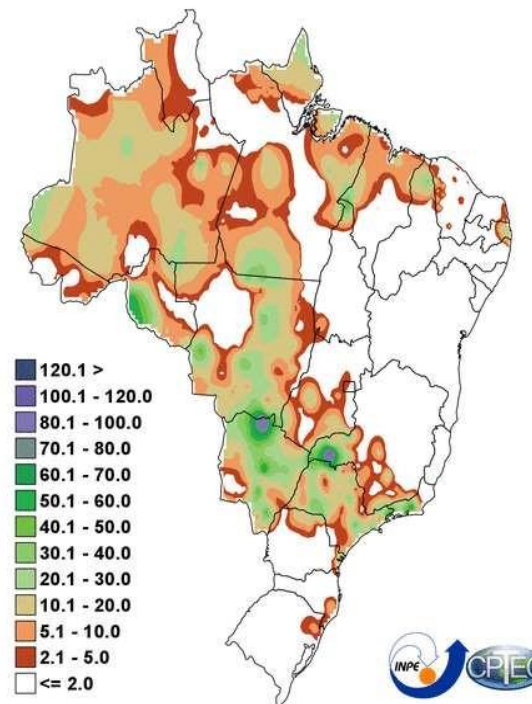
Precipitacao Observada (mm) - 13/02/2019
