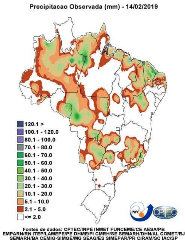
Figura 3 - Mapa de precipitação para os dias: (a) 12/02; (b) 13/02; e (c) 14/02.
