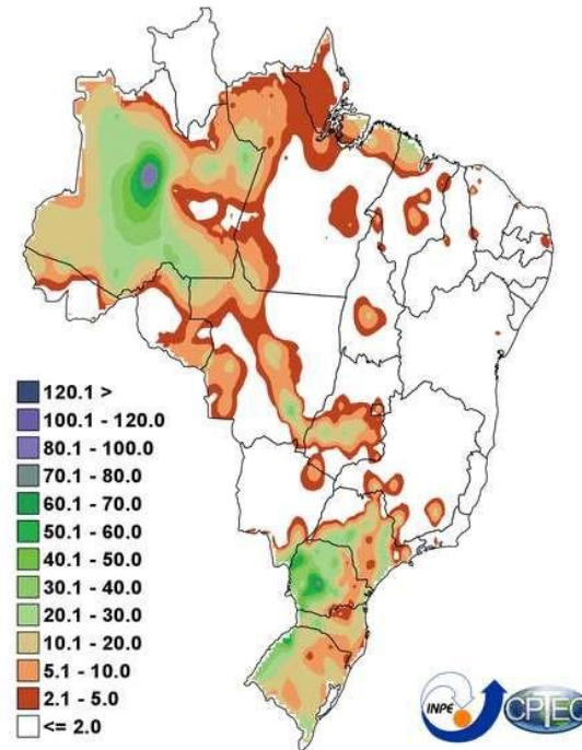
Precipitacao Observada (mm) - 12/02/2019
