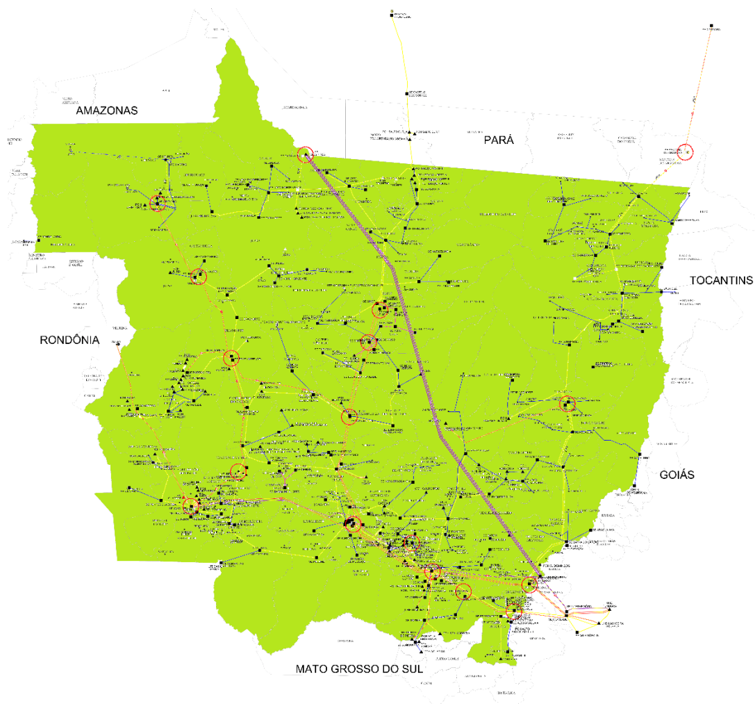
Figura 2 - Diagrama unifilar da subtransmissão com municípios do estado afetados pelos eventos.
