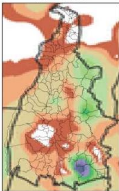
Mapa de Precipitação 2021-11-05
