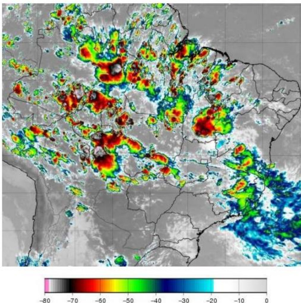
Figura 1 - Imagem de satélite no infravermelho com realce do satélite GOES-16 às 20:00 UT do dia 01/11. As cores indicam diferentes temperaturas dos topos das nuvens.
