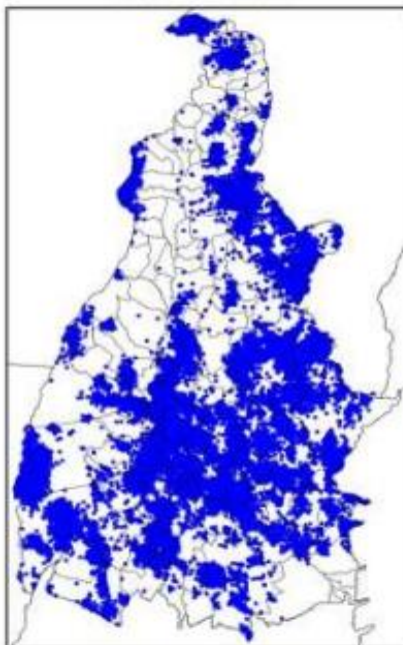
Mapa de Descargas Atmosféricas 2021-11-01
