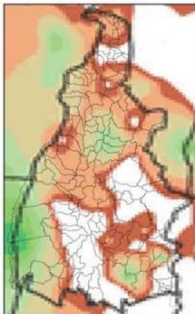
Mapa de Precipitação 2021-11-01
