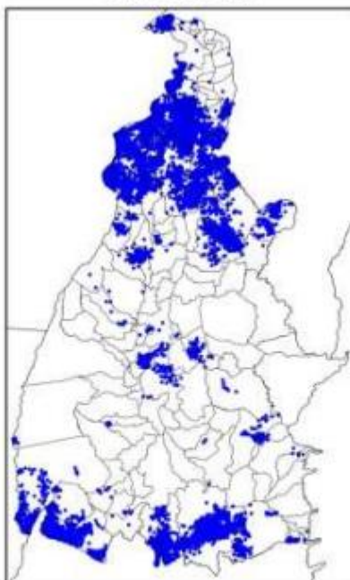
Mapa de Descargas Atmosféricas 2021-11-05
