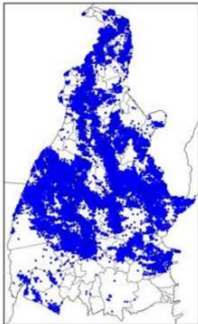
Mapa de Descargas Atmosféricas 2021-11-02
