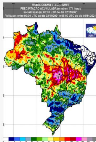
Figura 1: Previsão de acumulado de chuva entre os dias 02 e 09 de novembro de 2021. Fonte: INMET.
