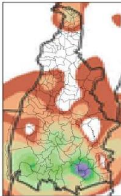
Mapa de Precipitação 2021-11-04
