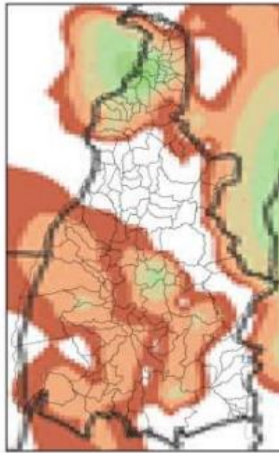
Mapa de Precipitação 2021-11-03
