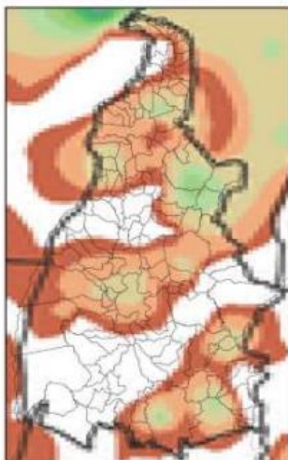
Mapa de Precipitação 2021-11-06
