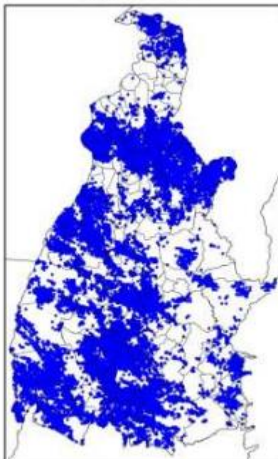
Mapa de Descargas Atmosféricas 2021-11-04
