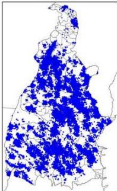
Mapa de Descargas Atmosféricas 2021-11-03
