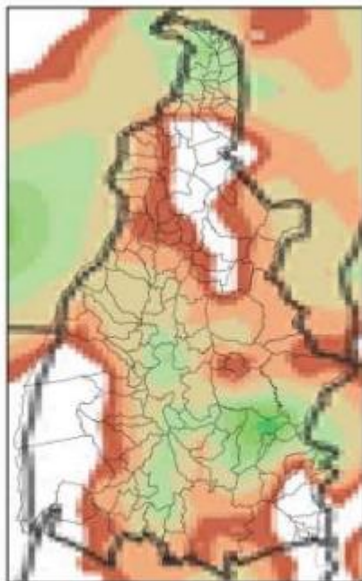
Mapa de Precipitação 2021-11-02
