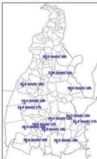
Mapa de Rajada Máxima 2021-11-06
