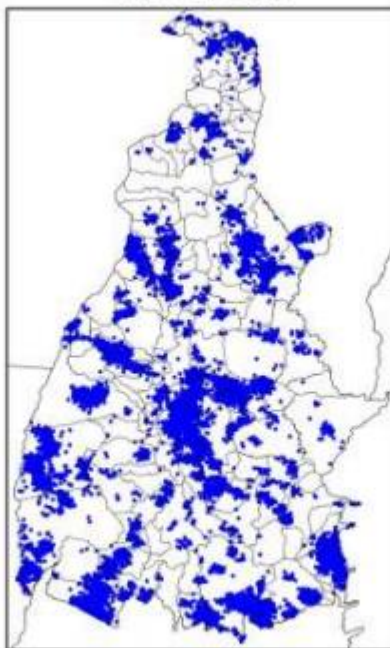
Mapa de Descargas Atmosféricas 2021-11-06
