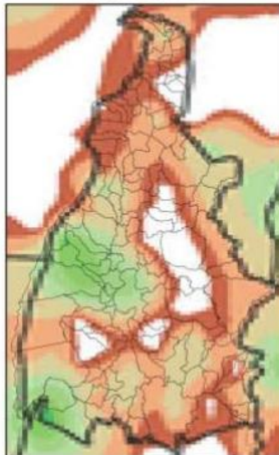
Mapa de Precipitação 2022-01-25
