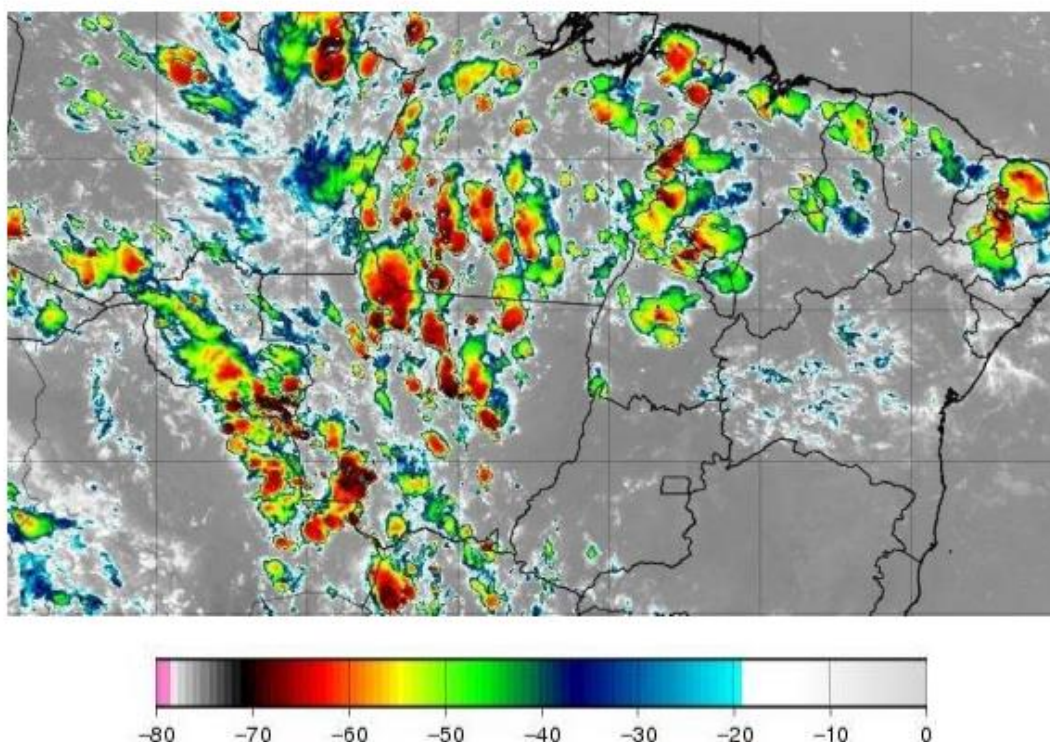
Figura 1 - Imagem de satélite no infravermelho com realce do satélite GOES-16 às 21:00 UT do dia 14/01. As cores indicam diferentes temperaturas dos topos das nuvens.
