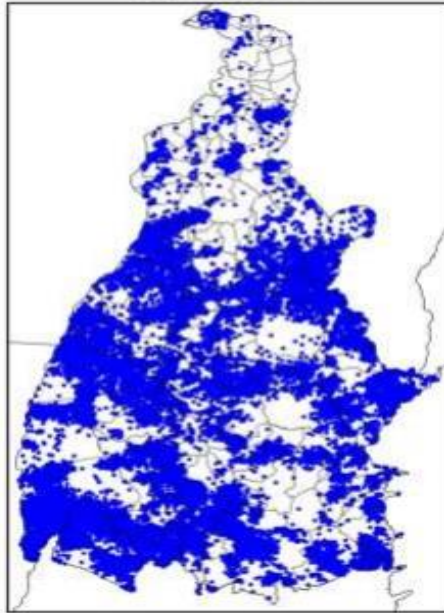
Mapa de Descargas Atmosféricas 2022-01-24
