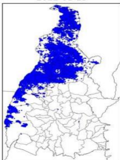
Mapa de Descargas Atmosféricas 2022-01-15
