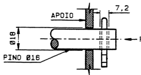
Figura 2 - Detalhe para execução do ensaio
