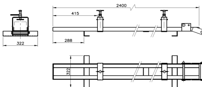
SUPORTE PARA CRUZETA
