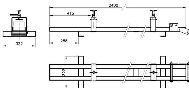
SUPORE PARA CRUZETA
