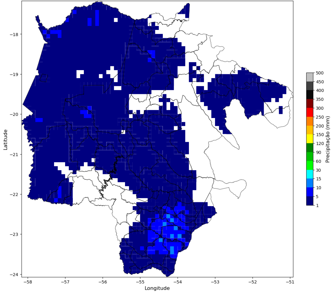
Precipitação no dia 2024-12-07 - EMS
