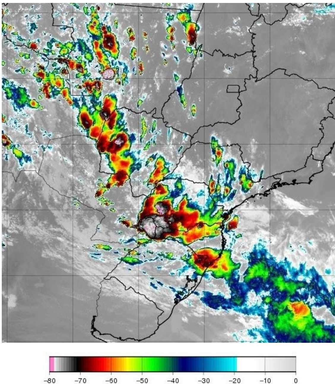
Figura 1 - Imagem de satélite no infravermelho com realce do satélite GOES-16 as 21:00 UT do dia 06/12. As cores indicam diferentes temperaturas dos topos das nuvens.
