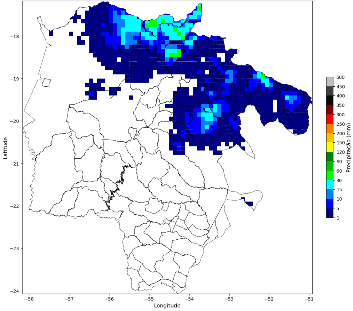
Precipitação no dia 2024-12-12 - EMS
