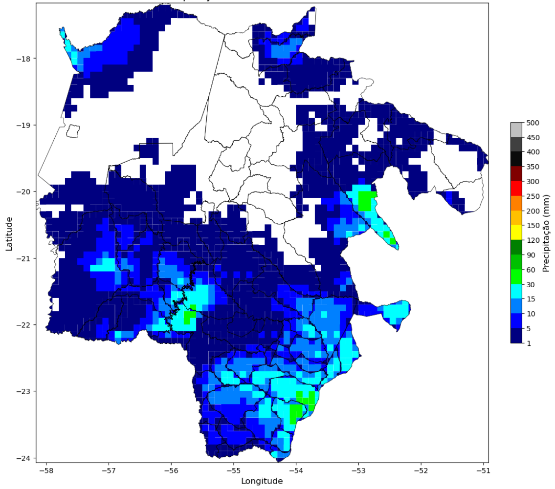
Precipitação no dia 2024-12-09 - EMS
