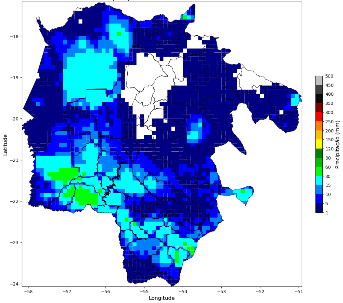
Precipitação no dia 2024-12-10 - EMS
