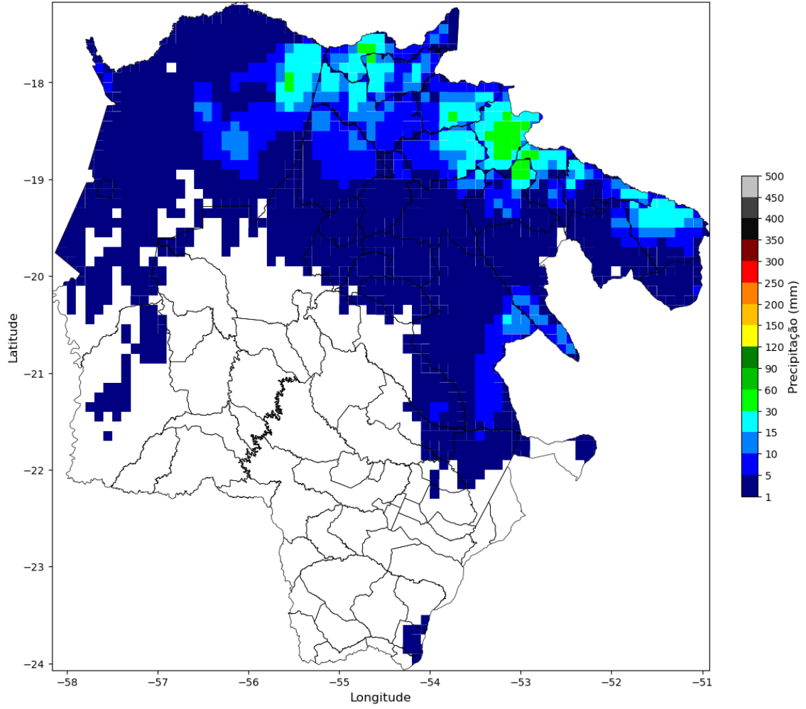
Precipitação no dia 2024-12-06 - EMS
