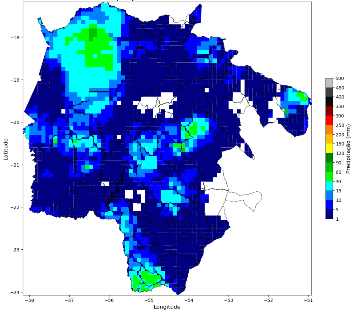
Precipitação no dia 2024-12-13 - EMS
