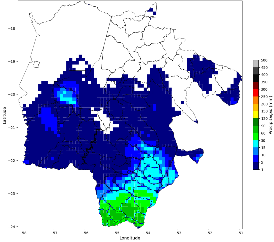
Precipitação no dia 2024-12-08 - EMS
