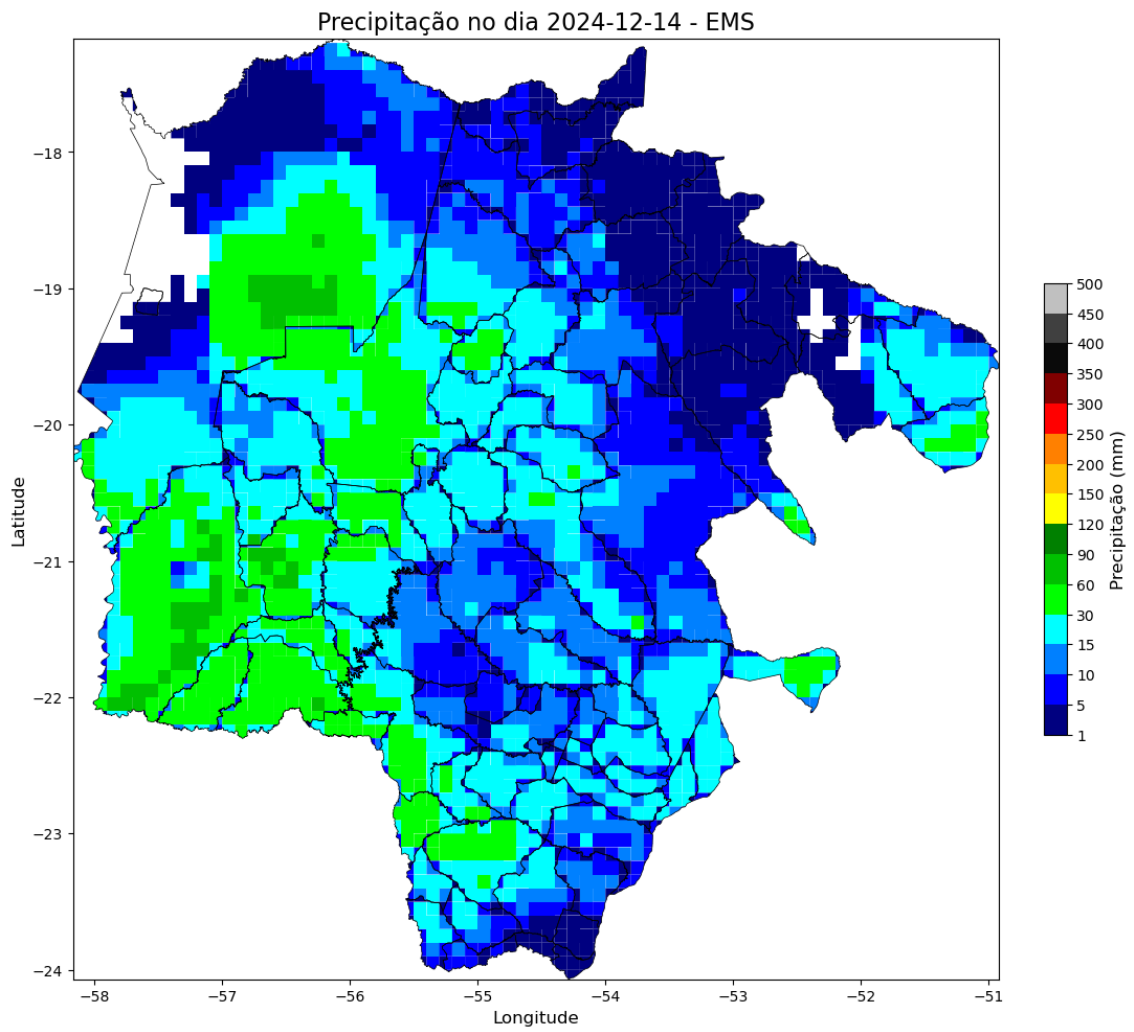
Figura 3 – Mapa de precipitação para os dias 06/12 a 14/12.
