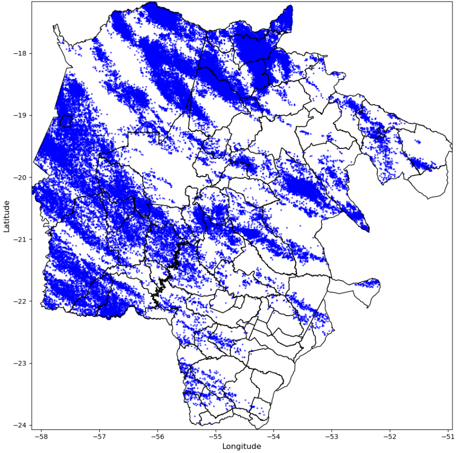
Descargas Atmosféricas - 2024-10-10
