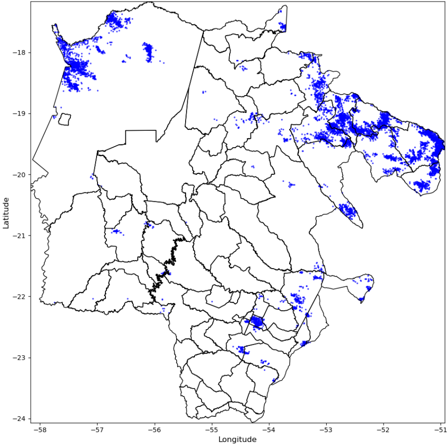
Descargas Atmosféricas - 2024-10-19
