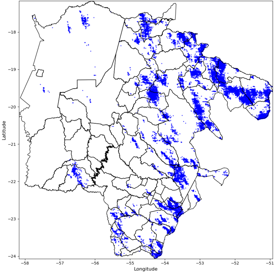
Descargas Atmosféricas - 2024-10-23
