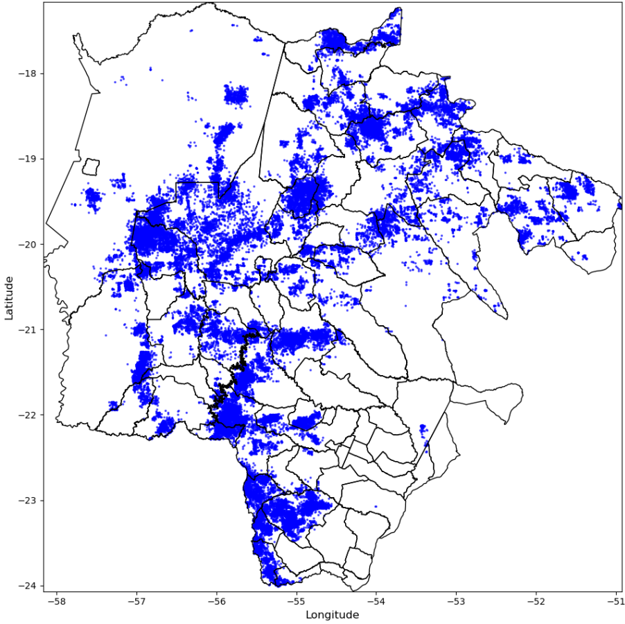
Descargas Atmosféricas - 2024-10-17
