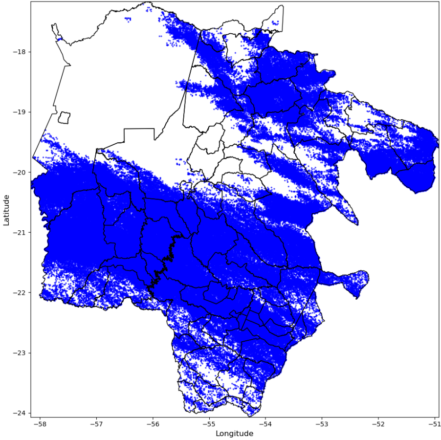
Descargas Atmosféricas - 2024-10-11
