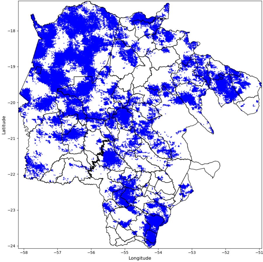
Descargas Atmosféricas - 2024-10-18
