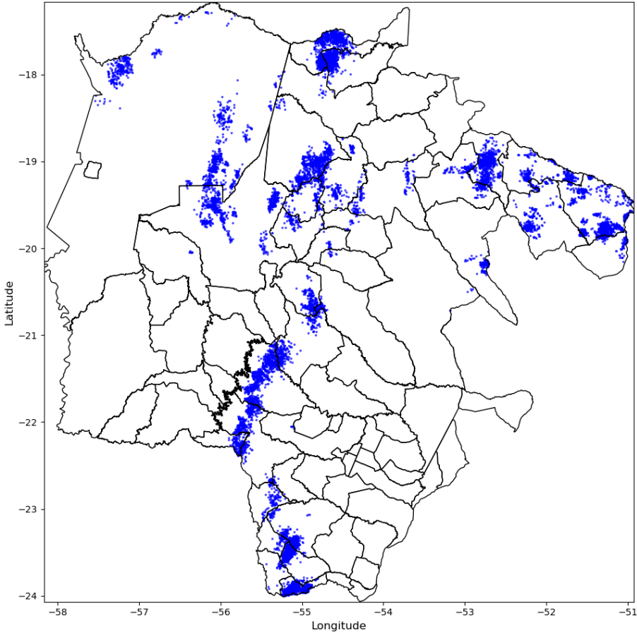
Descargas Atmosféricas - 2024-10-15
