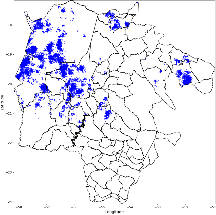
Descargas Atmosféricas - 2024-10-21
