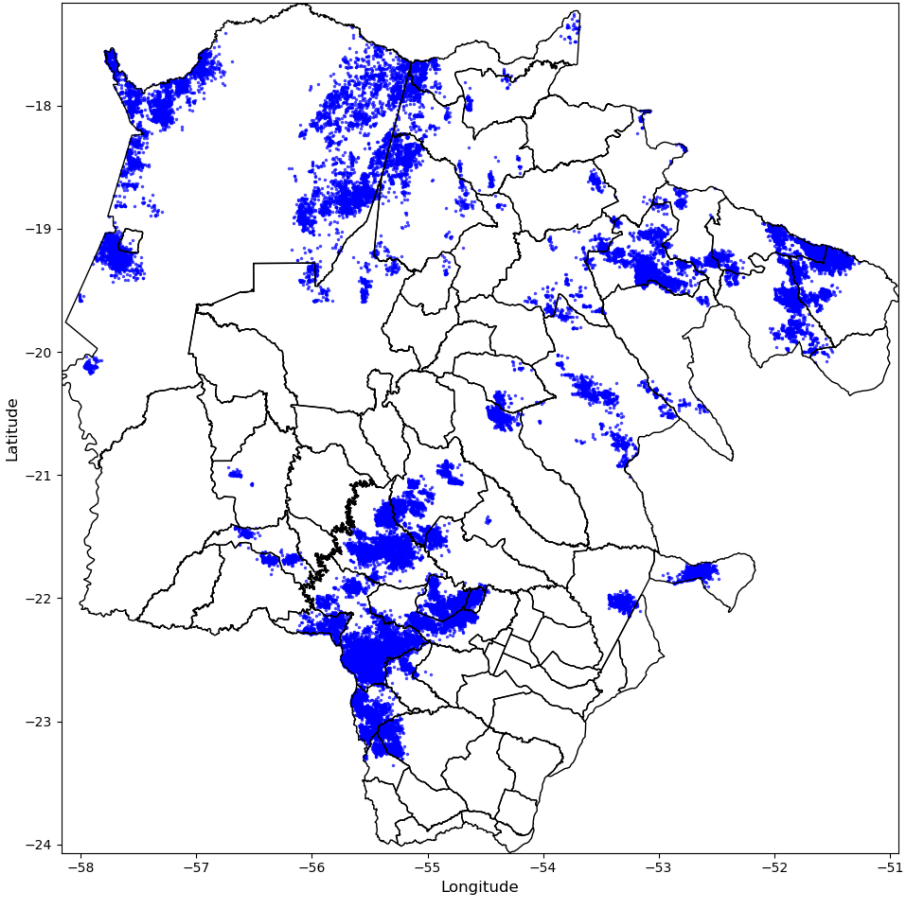
Descargas Atmosféricas - 2024-10-16
