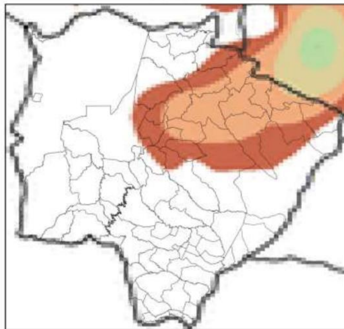
Mapa de Precipitação 2023-10-16
