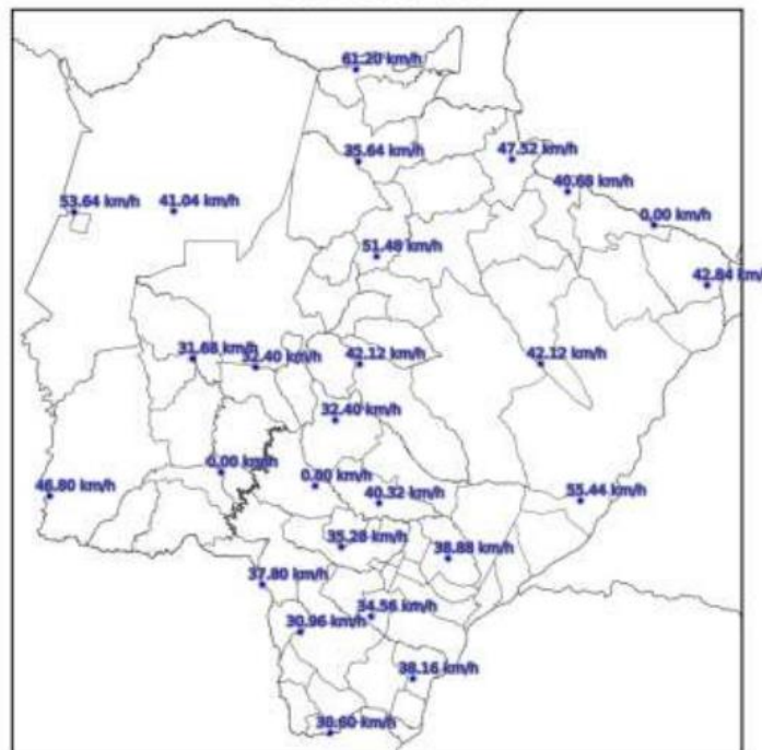
Mapa de Rajada Máxima 2023-10-12
