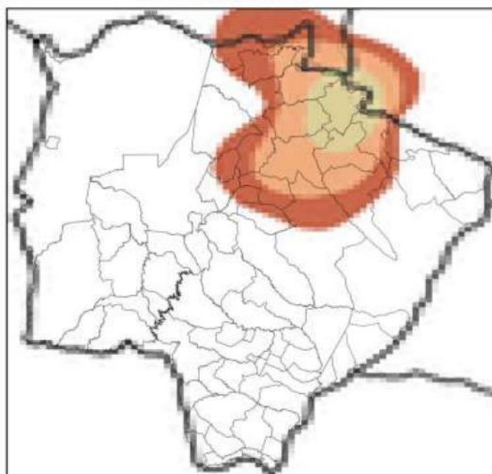
Mapa de Precipitação 2023-10-15
