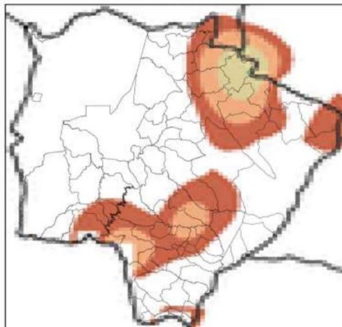
Mapa de Precipitação 2023-10-21
