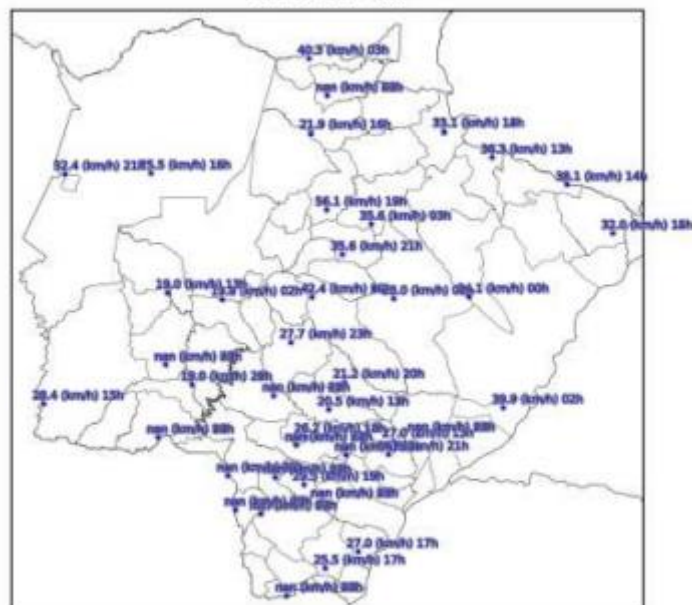
Mapa de Rajada Máxima 2022-10-16
