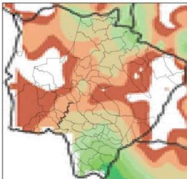
Mapa de Precipitação 2022-10-12
