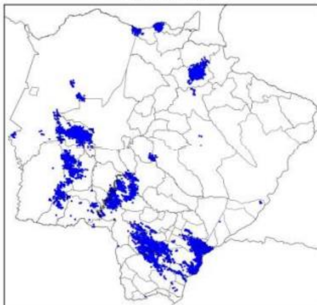
Mapa de Descargas Atmosféricas 2022-10-14
