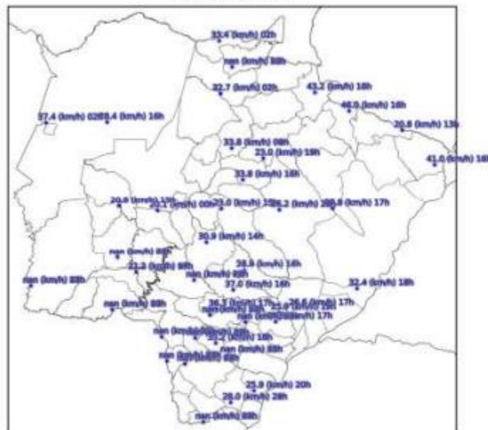
Mapa de Rajada Máxima 2022-10-10
