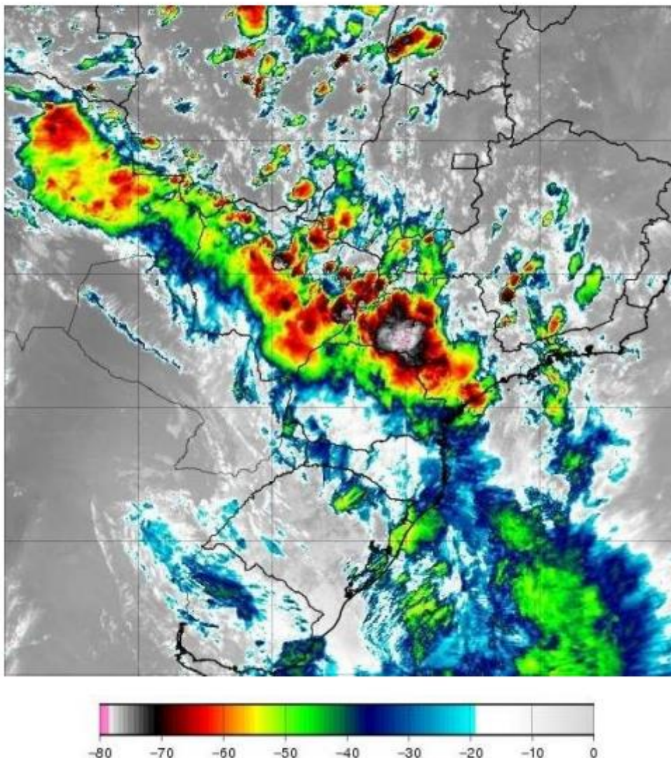
Figura 1 - Imagem de satélite no infravermelho com realce do satélite GOES-16 as 21:00 UT do dia 06/10. As cores indicam diferentes temperaturas dos topos das nuvens.
