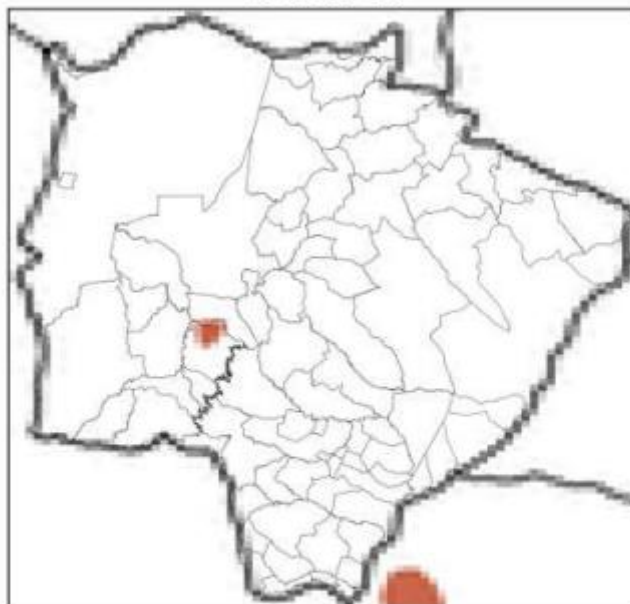
Mapa de Precipitação 2022-10-16
