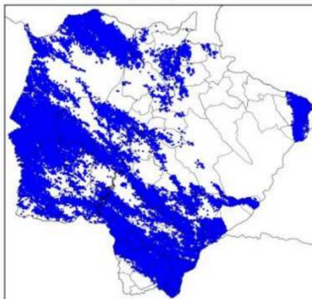
Mapa de Descargas Atmosféricas 2022-10-12
