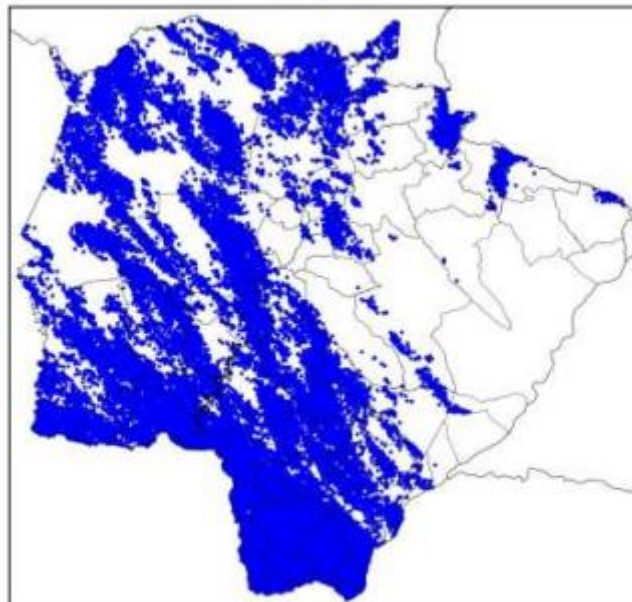
Mapa de Descargas Atmosféricas 2022-10-11
