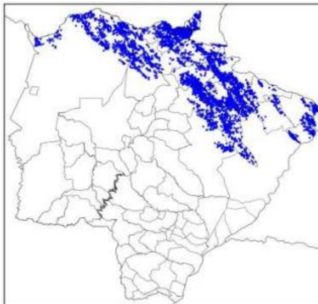
Mapa de Descargas Atmosféricas 2022-10-07
