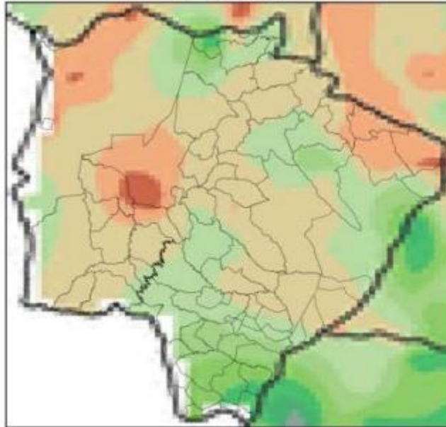
Mapa de Precipitação 2022-10-07
