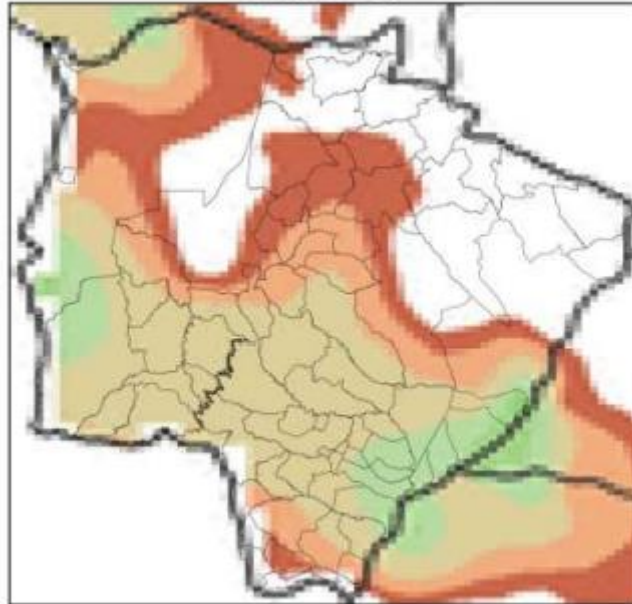
Mapa de Precipitação 2022-10-13
