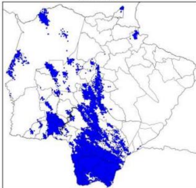
Mapa de Descargas Atmosféricas 2022-10-13
