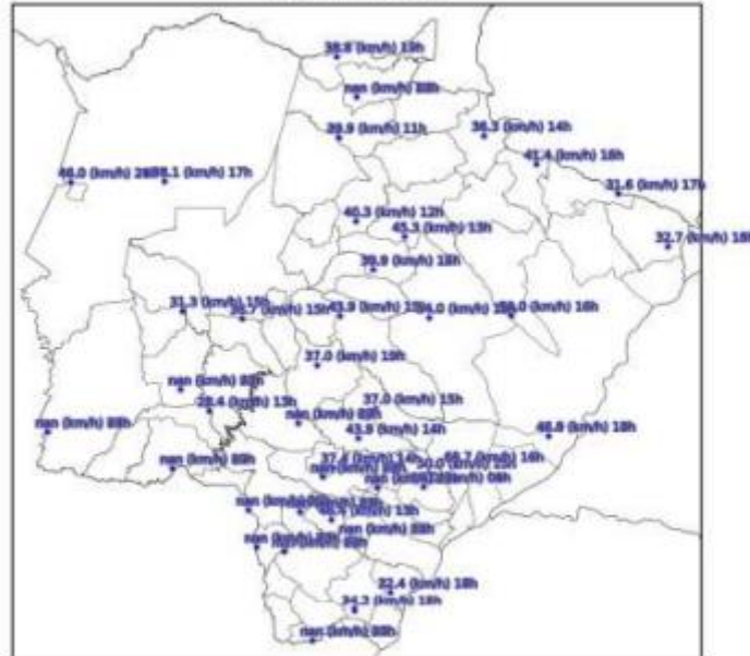
Mapa de Rajada Máxima 2022-10-09
