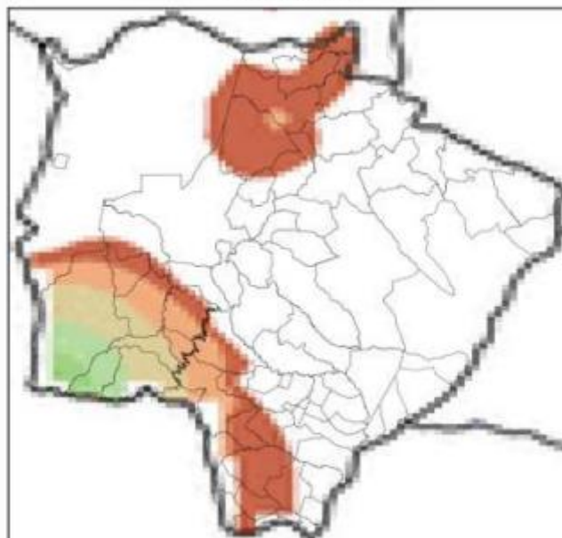
Mapa de Precipitação 2022-10-09
