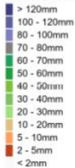
Figura 3 – Mapa de precipitação para os dias: (a) 06/10; (b) 07/10; (c) 08/10; (d) 09/10; (e) 10/10; (f) 11/10; (g) 12/10; (h) 13/10; (i) 14/10; (j) 15/10; e (k) 16/10.
