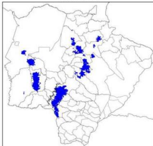
Mapa de Descargas Atmosféricas 2022-10-16
