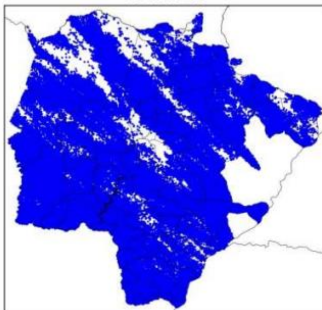
Mapa de Descargas Atmosféricas 2022-10-06
