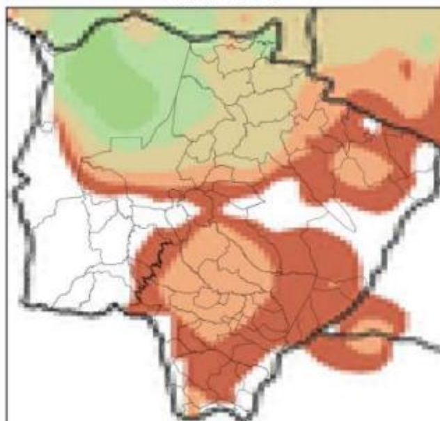
Mapa de Precipitação 2022-10-10
