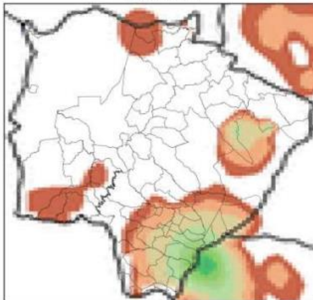
Mapa de Precipitação 2022-10-11
