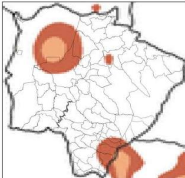
Mapa de Precipitação 2022-10-15
