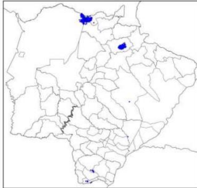
Mapa de Descargas Atmosféricas 2022-10-15
