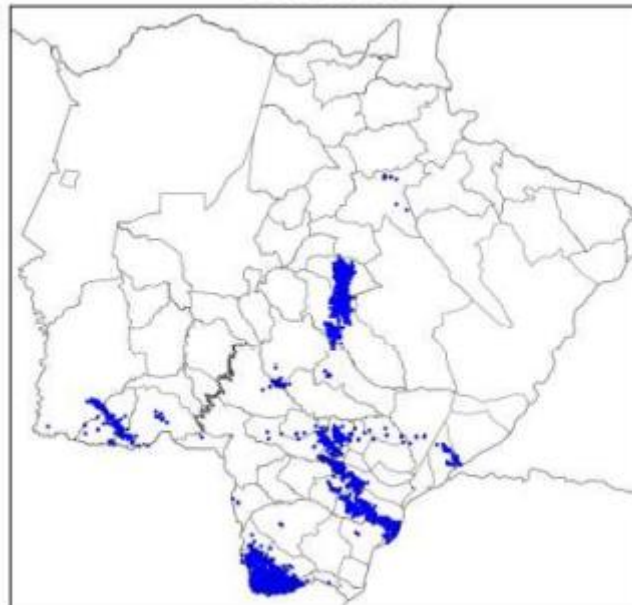
Mapa de Descargas Atmosféricas 2022-10-10
