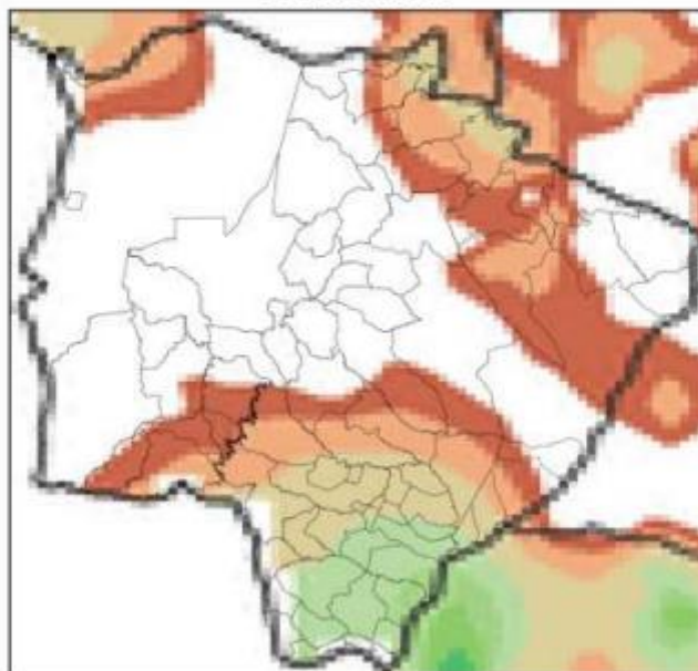
Mapa de Precipitação 2022-10-06
