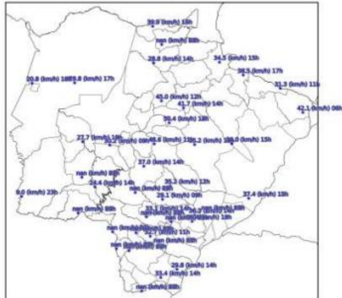
Mapa de Rajada Máxima 2022-10-15
