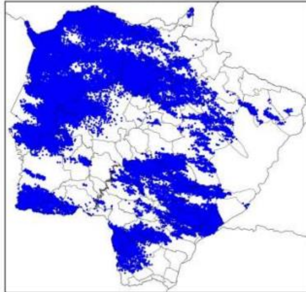
Mapa de Descargas Atmosféricas 2022-10-09
