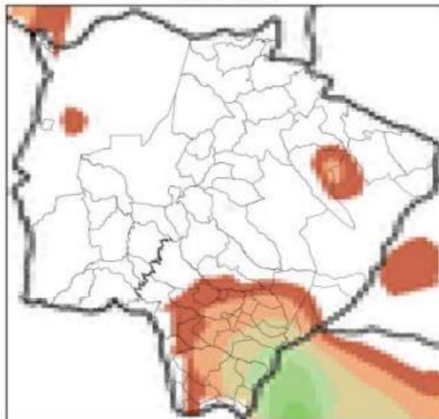
Mapa de Precipitação 2022-10-14
