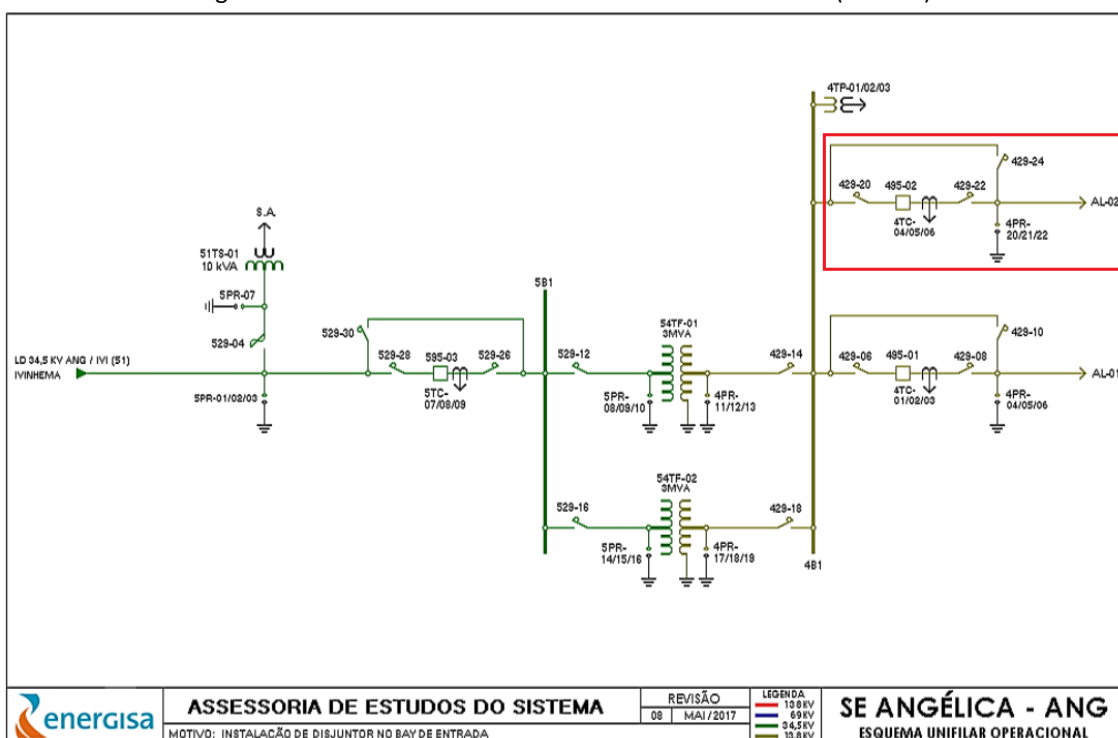
Figura 4 - Alimentadores afetados circulos em vermelho (SE ANG).
