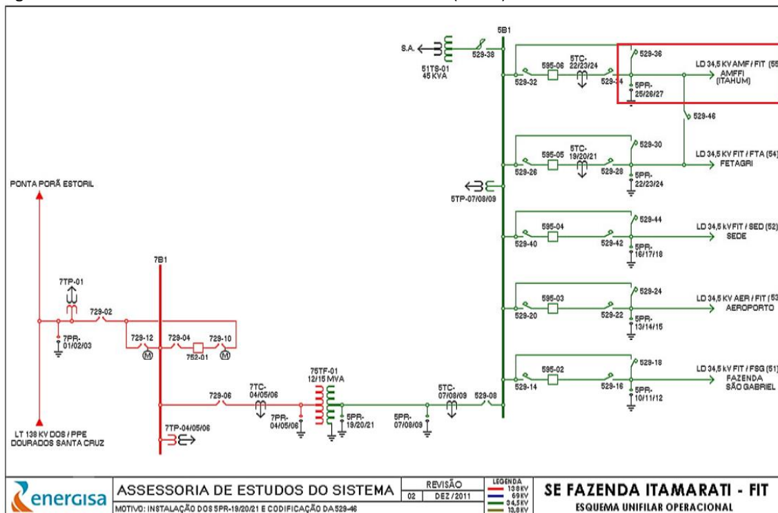
Figura 10 - Alimentadores afetados circulados em vermelho (SE FIT).
