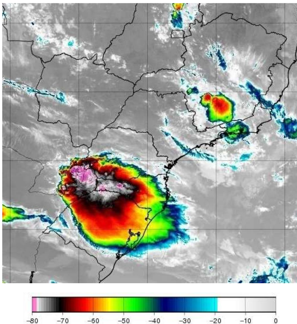
Figura 1 - Imagem de satélite no infravermelho com realçado satélite GOES-16 durante
