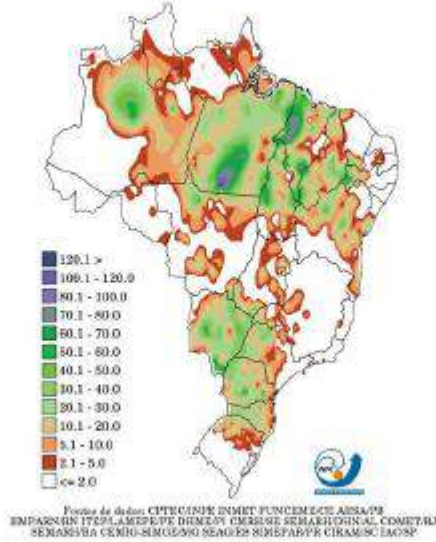
Precipitação Observada (mm) - 14/04/2020
