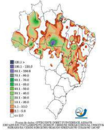
Precipitação Observada (mm) - 16/04/2020
