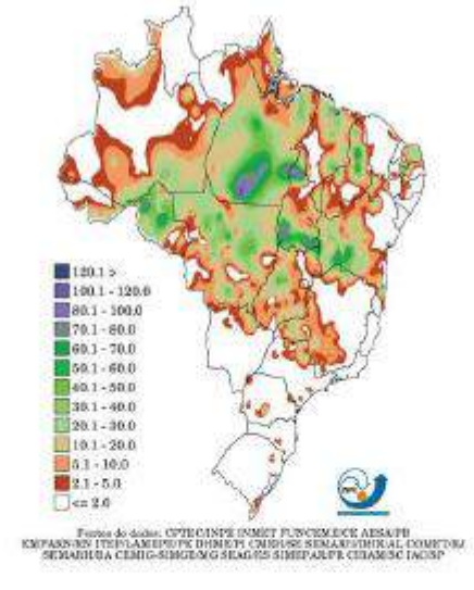
Precipitação Observada (mm) - 15/04/2020
