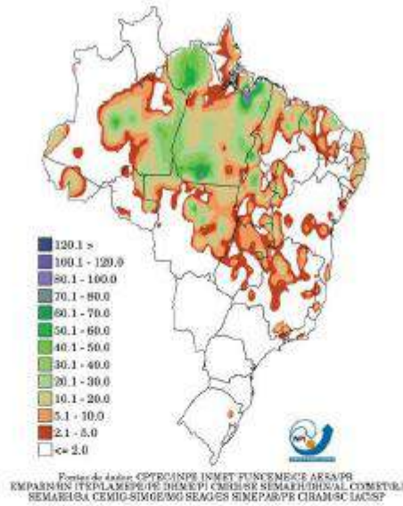
Precipitação Observada (mm) - 17/04/2020
