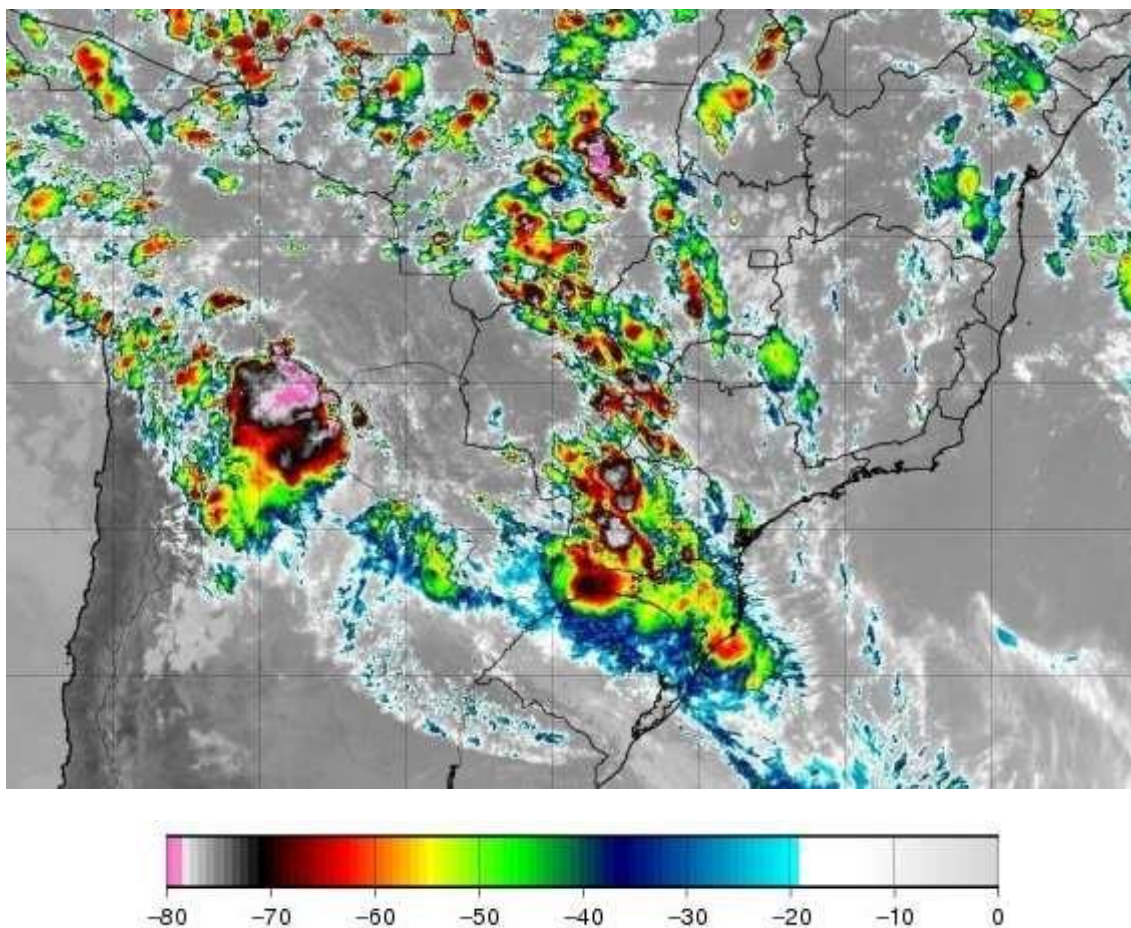
Figura 1 - Imagem de satélite no infravermelho com realce do satélite GOES-16 as 20:00 UT do dia 18/02. As cores indicam diferentes temperaturas dos topos das nuvens.
