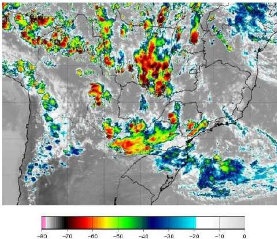
Figura 1 - Imagem de satélite no infravermelho com realce do satélite GOES-16 durante um dos períodos de máxima intensidade do evento às 21:00 UT do dia 22/01. As cores indicam diferentes temperaturas dos topos das nuvens.
