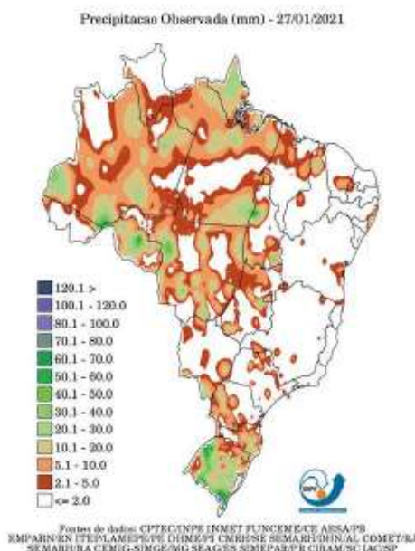
Figura 3 – Mapa de precipitação para os dias: (a) 22/01; (b) 23/01; (c) 24/01; (d) 25/01; (e) 26/01; e (f) 27/01.
