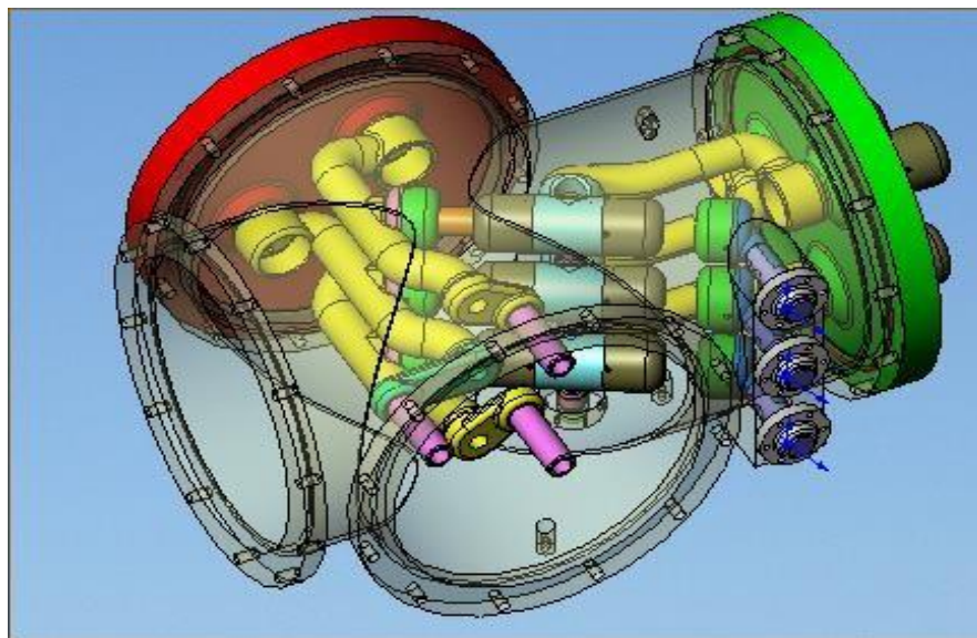
Figura 13: Vista isométrica chave seccionadora de três posições
