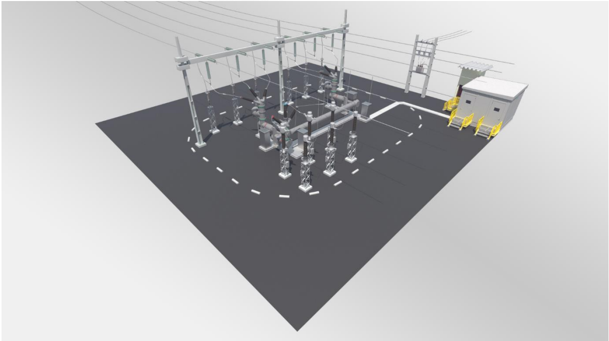
Figura 8: Modelo 3D - SED Tipo 05 vista isométrica com TC e TP
