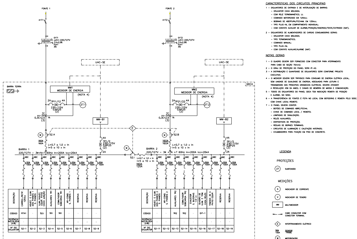
Figura 21 - Diagrama unifilar do painel QDCA com duas barras
