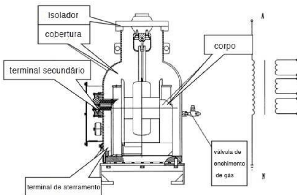
Figura 15: Modelo do módulo de transformador de potencial
