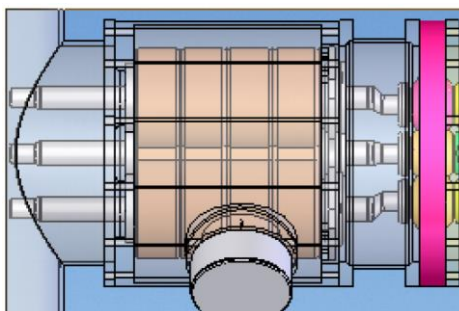
Figura 14: Modelo do módulo de transformador de corrente
