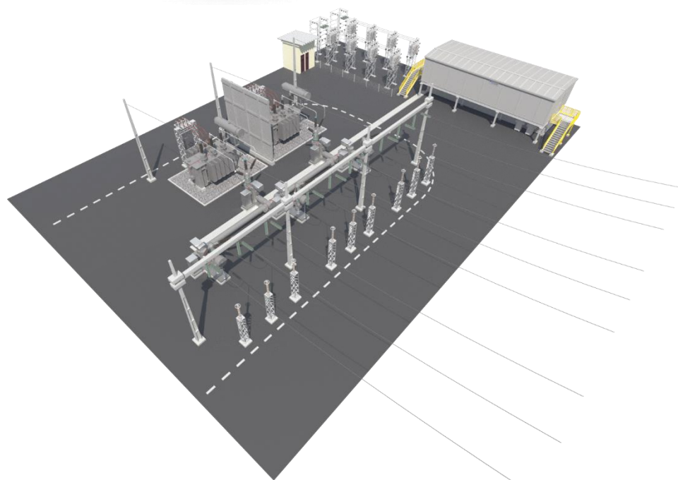
Figura 3: Modelo 3D - SED Tipo 02 vista isométrica
