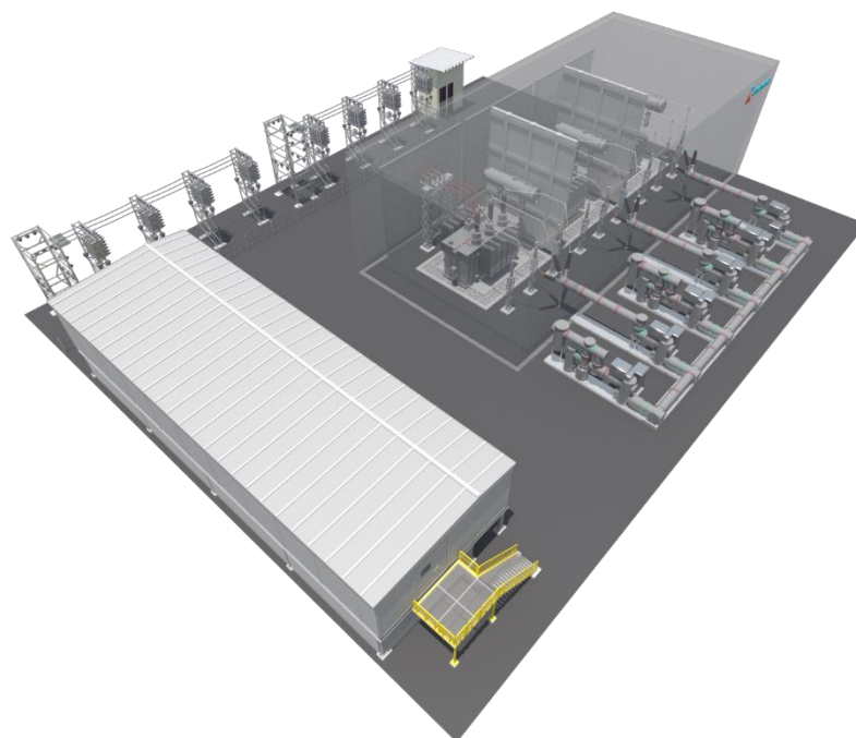
Figura 6: Modelo 3D - SED Tipo 04 vista isométrica
