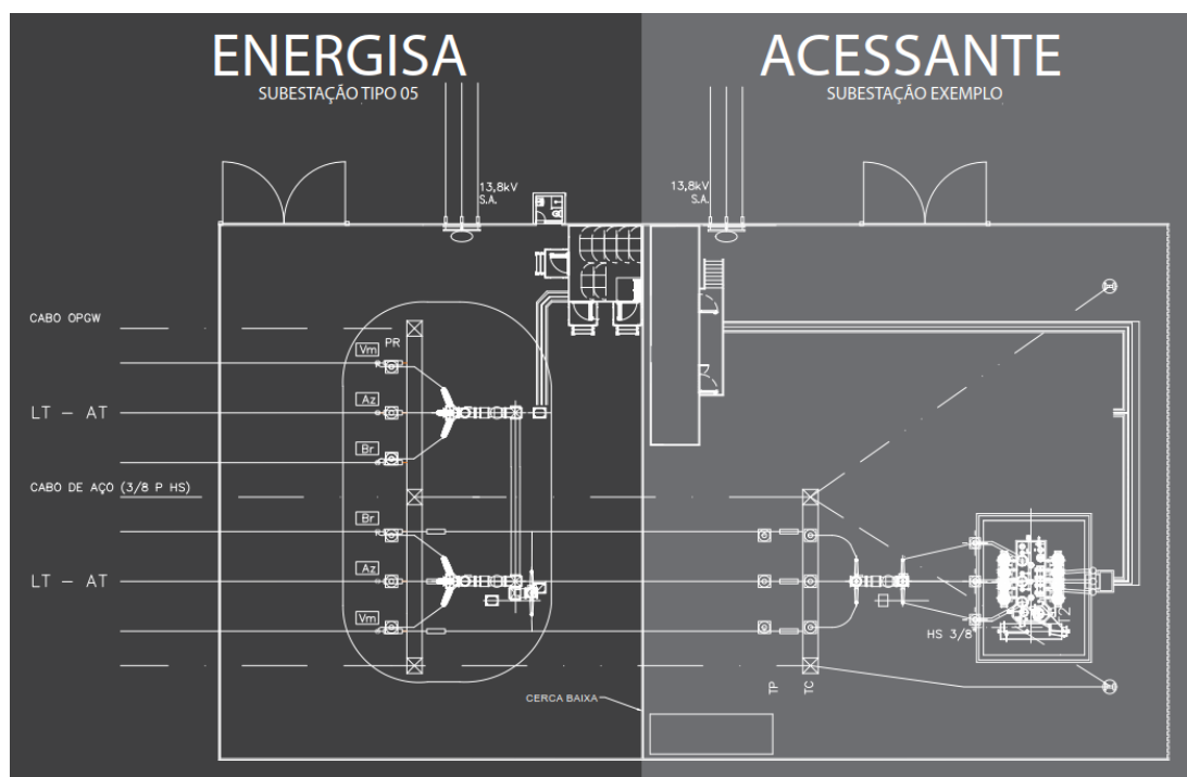
Figura 7: Exemplo de aplicação da SED Tipo 05
