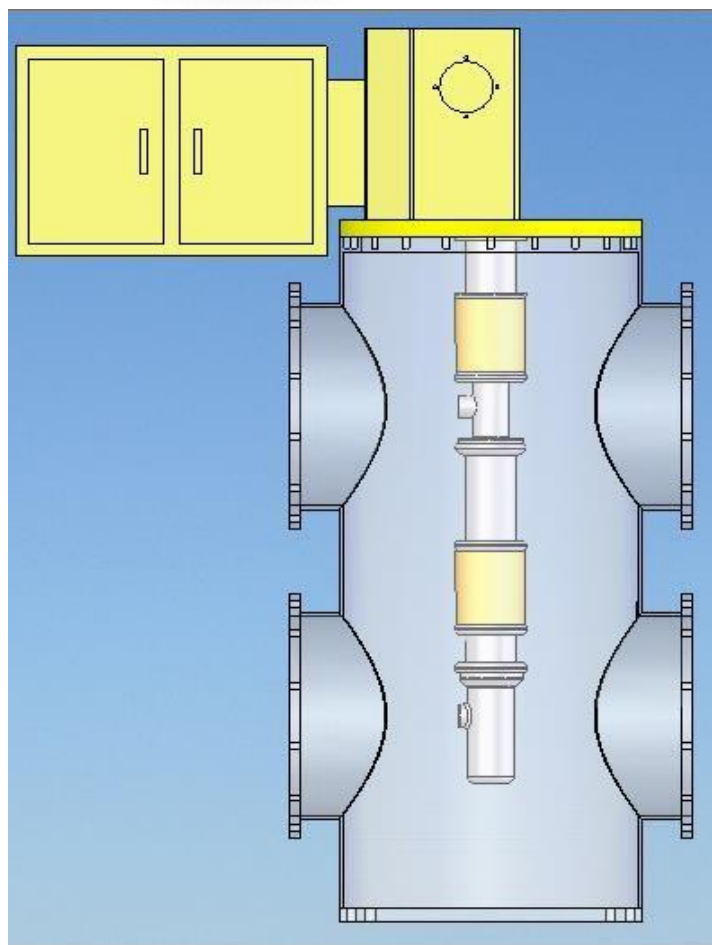
Figura 12: Estrutura do compartimento do disjuntor (GCB)
