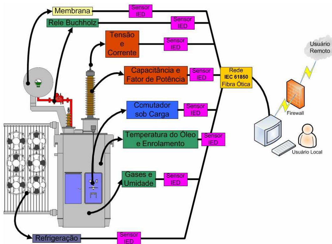
Figura 27 - Arquitetura do sistema descentralizado de aquisição e monitoramento.
