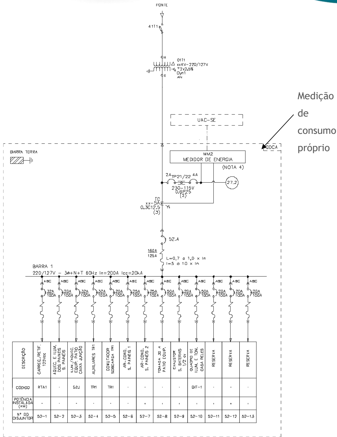
Figura 25: Diagrama Unifilar QDCA - uma entrada
