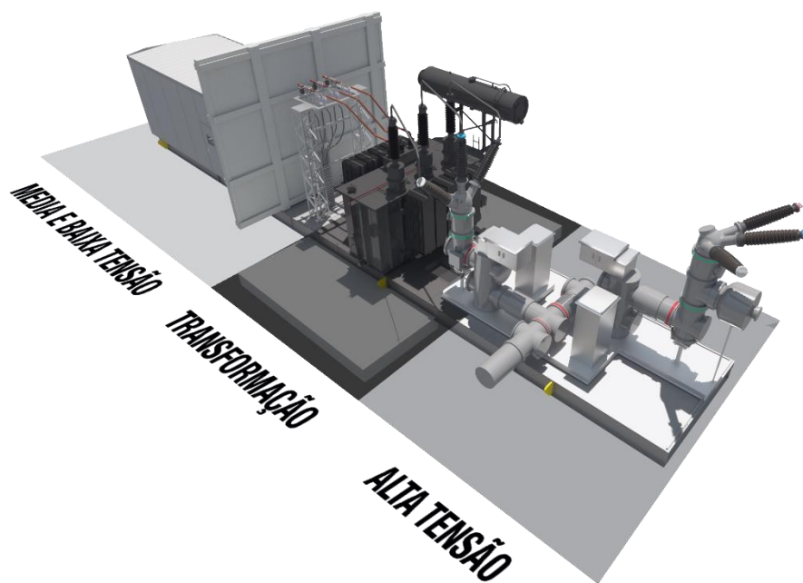
Figura 1: CMI composto por alta tensão, transformação e média e baixa tensão
