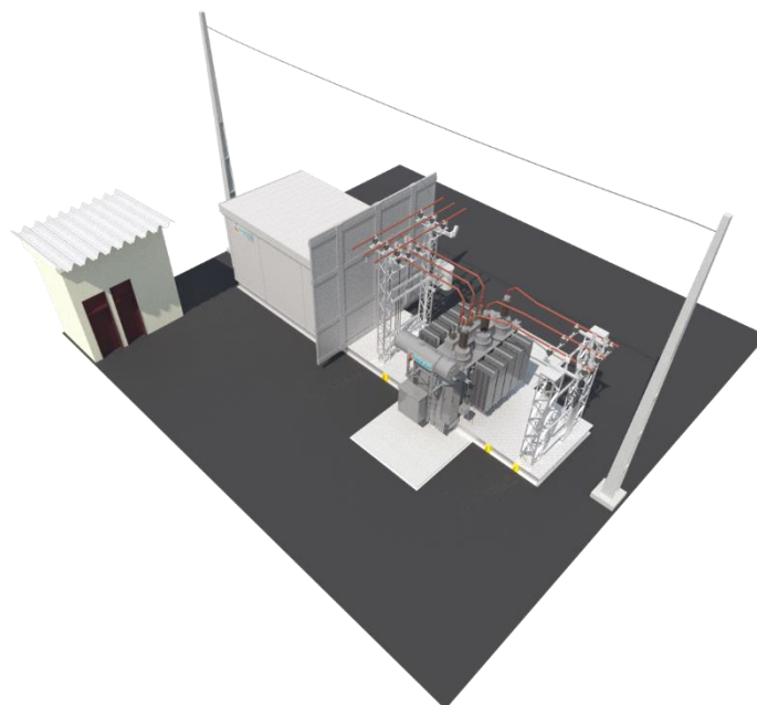
Figura 5: Modelo 3D - SED Tipo 03 vista em perspectiva
