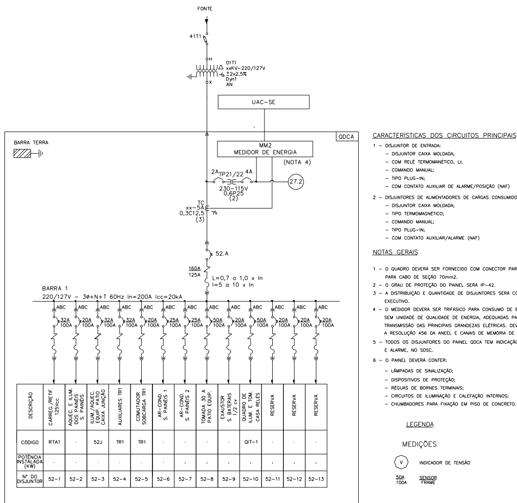
Figura 20 - Diagrama unifilar do painel QDCA com barra única
