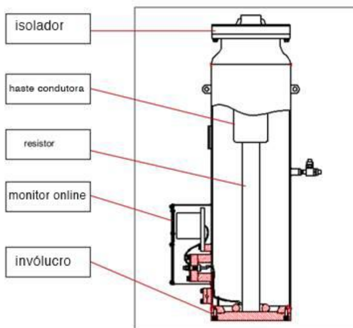
Figura 16: Modelo do módulo de transformador de corrente
