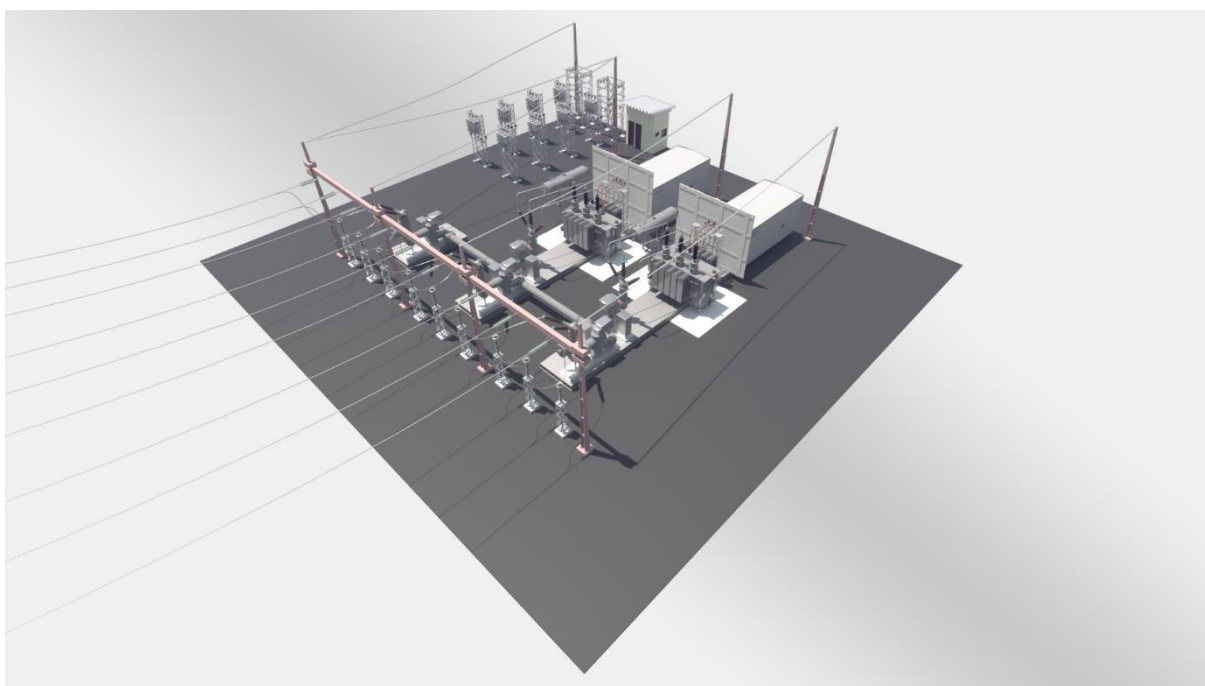
Figura 2: Modelo 3D - SED Tipo 01 vista isométrica
