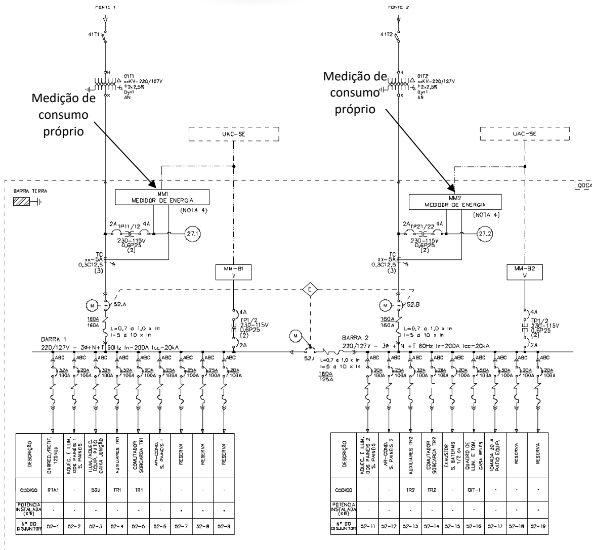
Figura 26: Diagrama Unifilar QDCA - duas entradas
