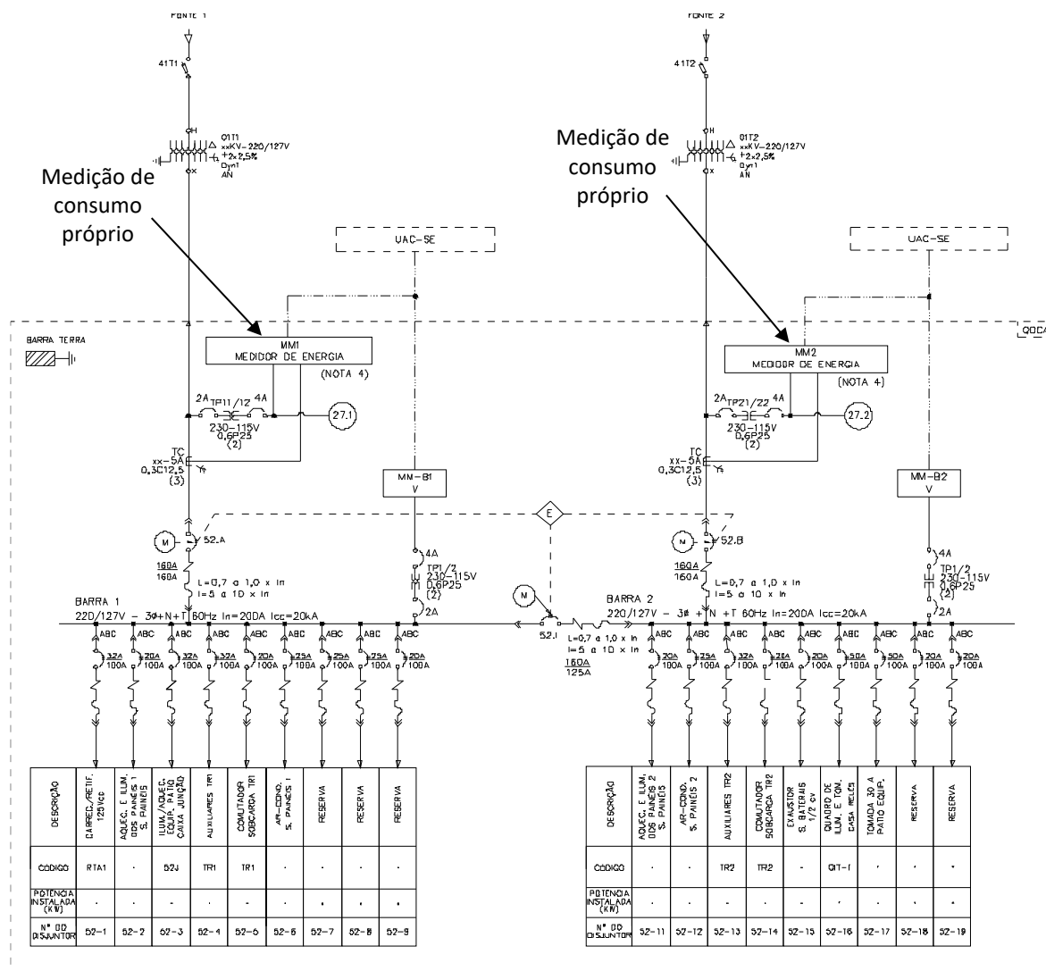
Figura 22 - Diagrama Unifilar QDCA - duas entradas
