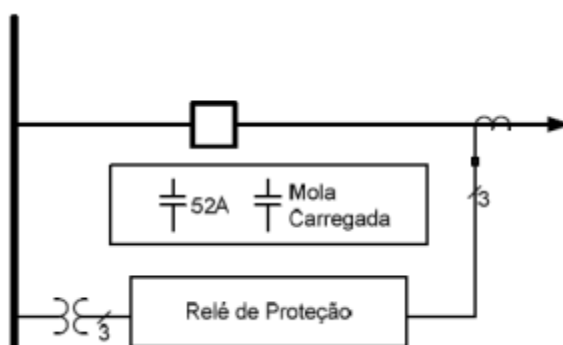
Figura 27 - Diagrama básico de conexão para monitoramento de disjuntores
