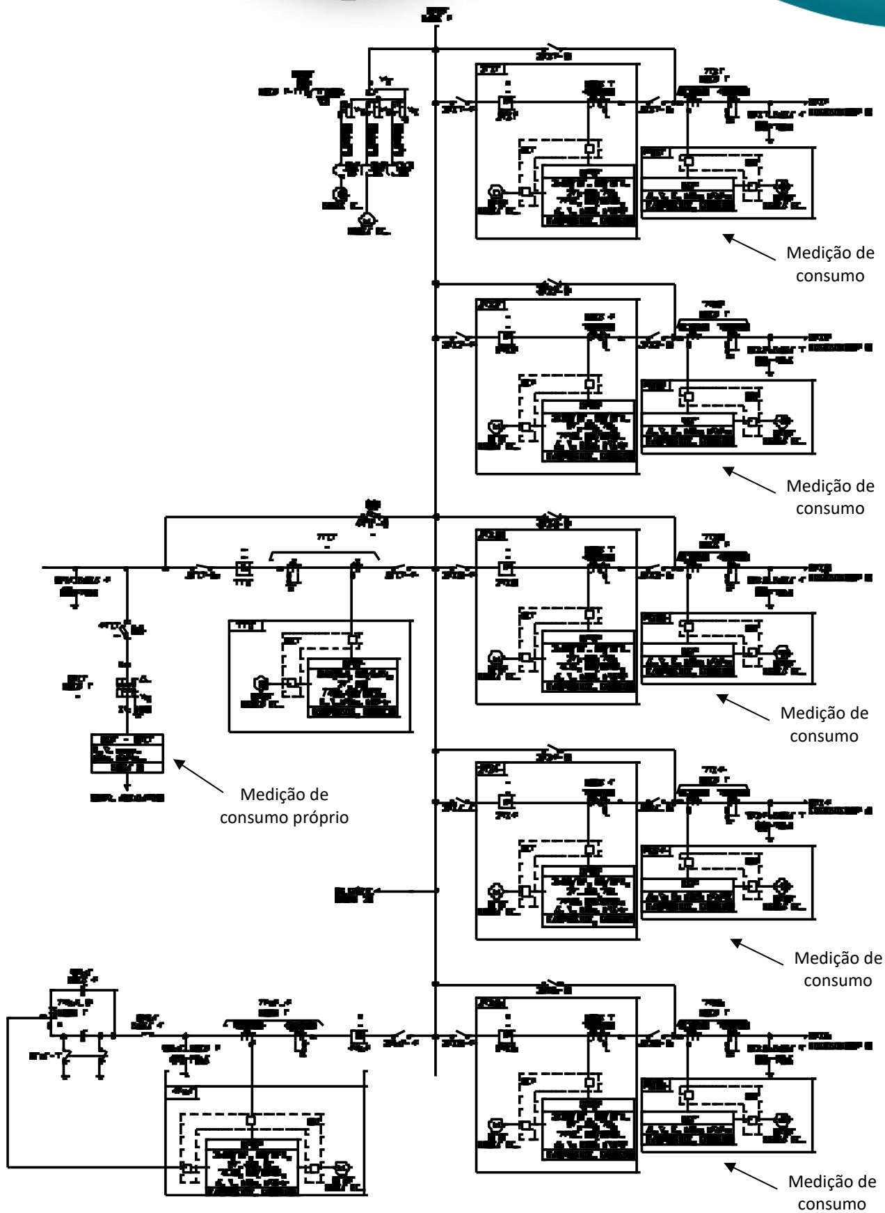
Figura 25 - Diagrama unifilar do setor de MT.
