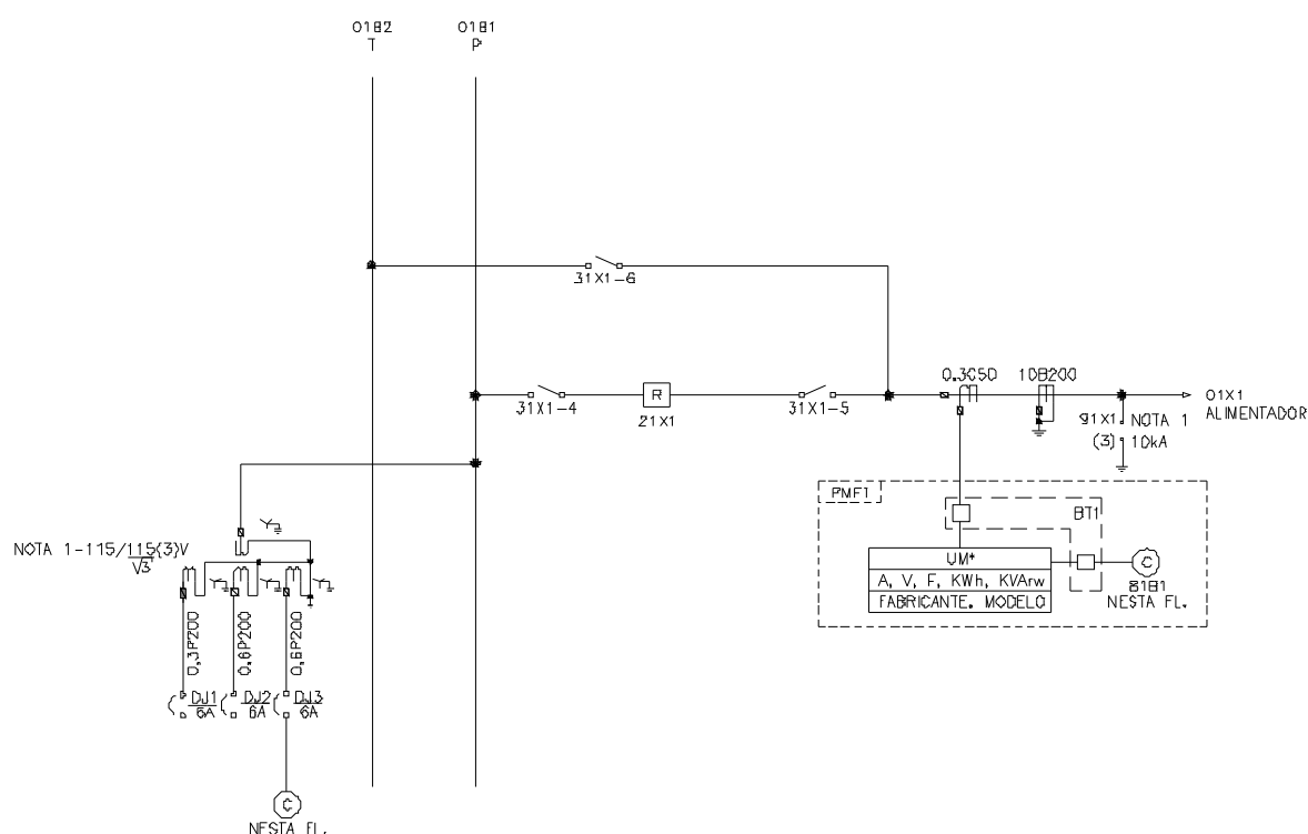
Figura 19 - Diagrama unifilar mostrando a ligação dos medidores de consumo.
