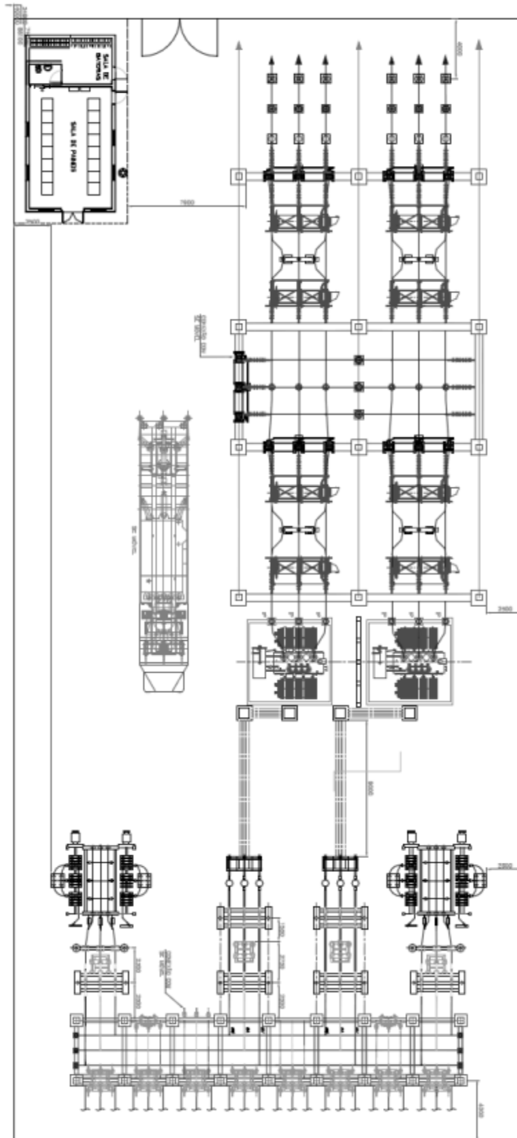
Figura 5: Subestação tipo Rural 4 (barramento simples na AT e barramento simples na MT).
