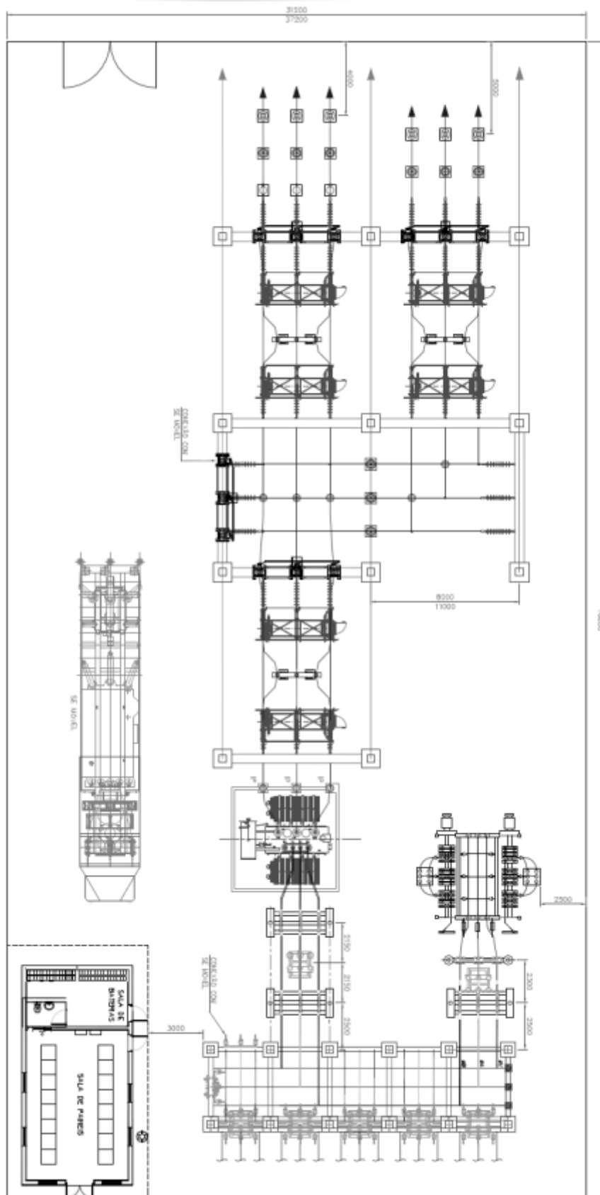
Figura 3: Subestação tipo Rural 2 (barramento simples na AT e barramento simples na MT).
