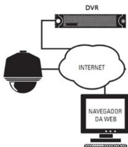
Figura 28 - Arquitetura do sistema CFTV proposto.
