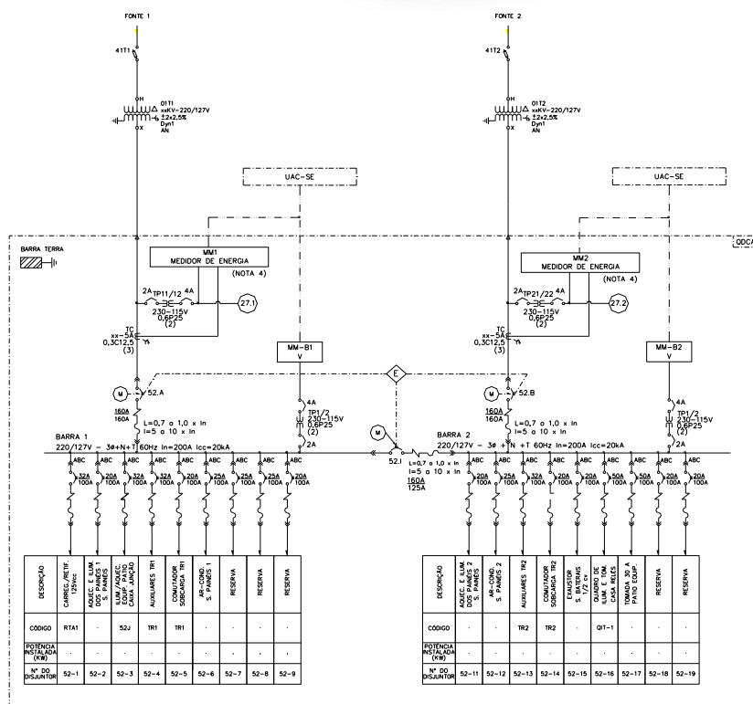
Figura 16 - Diagrama unifilar do painel QDCA com duas barras
