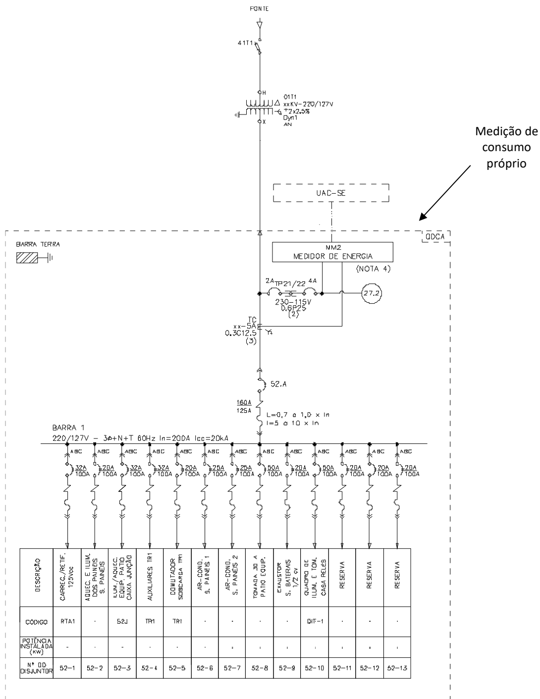
Figura 21 - Diagrama Unifilar QDCA - uma entrada
