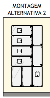
VISTA FRONTAL EXTERNO 1 : 50
