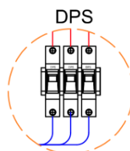
DETALHE A
