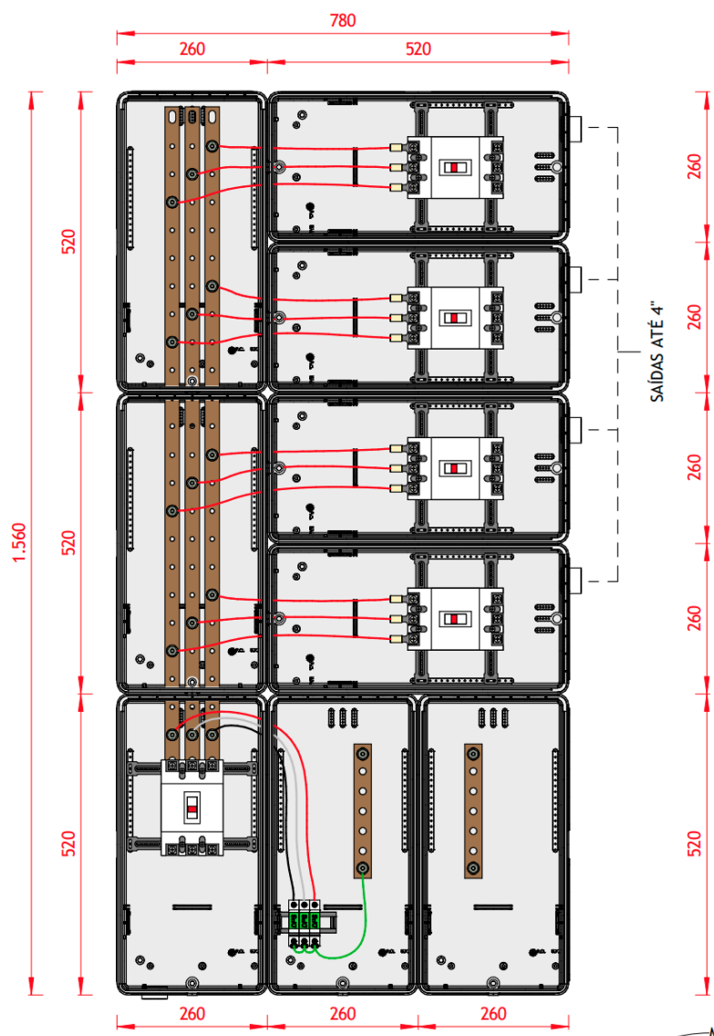
VISTA FRONTAL INTERNO 1 : 10
