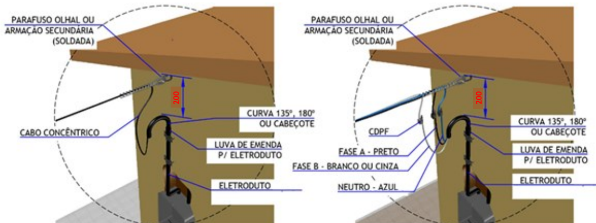
DETALHE A - TIPO LIGAÇÃO: MONOFÁSICO ESC.: N.I.
