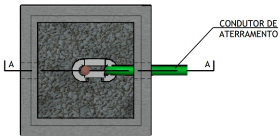
VISTA EM PLANTA - SEM TAMPA ESC.: 1/5
