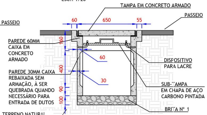
VISTA EM CORTE B ESC.: 1/20
