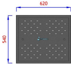
VISTA EM PLANTA - TAMPA METAL EXTERNA ESC.: 1/20
