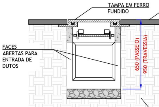
VISTA EM CORTE A ESC.: 1/20
