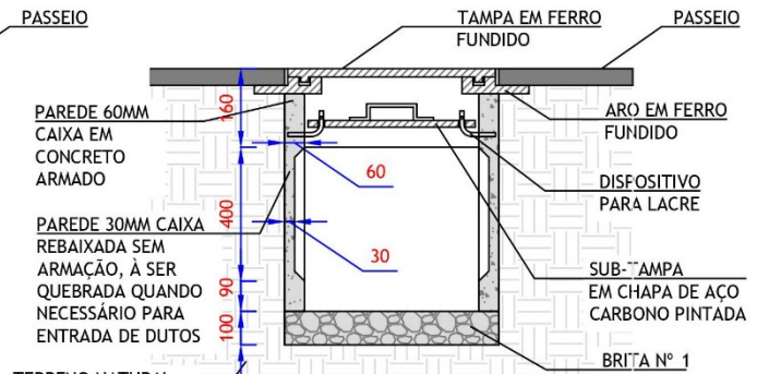
VISTA EM CORTE B ESC.: 1/20
