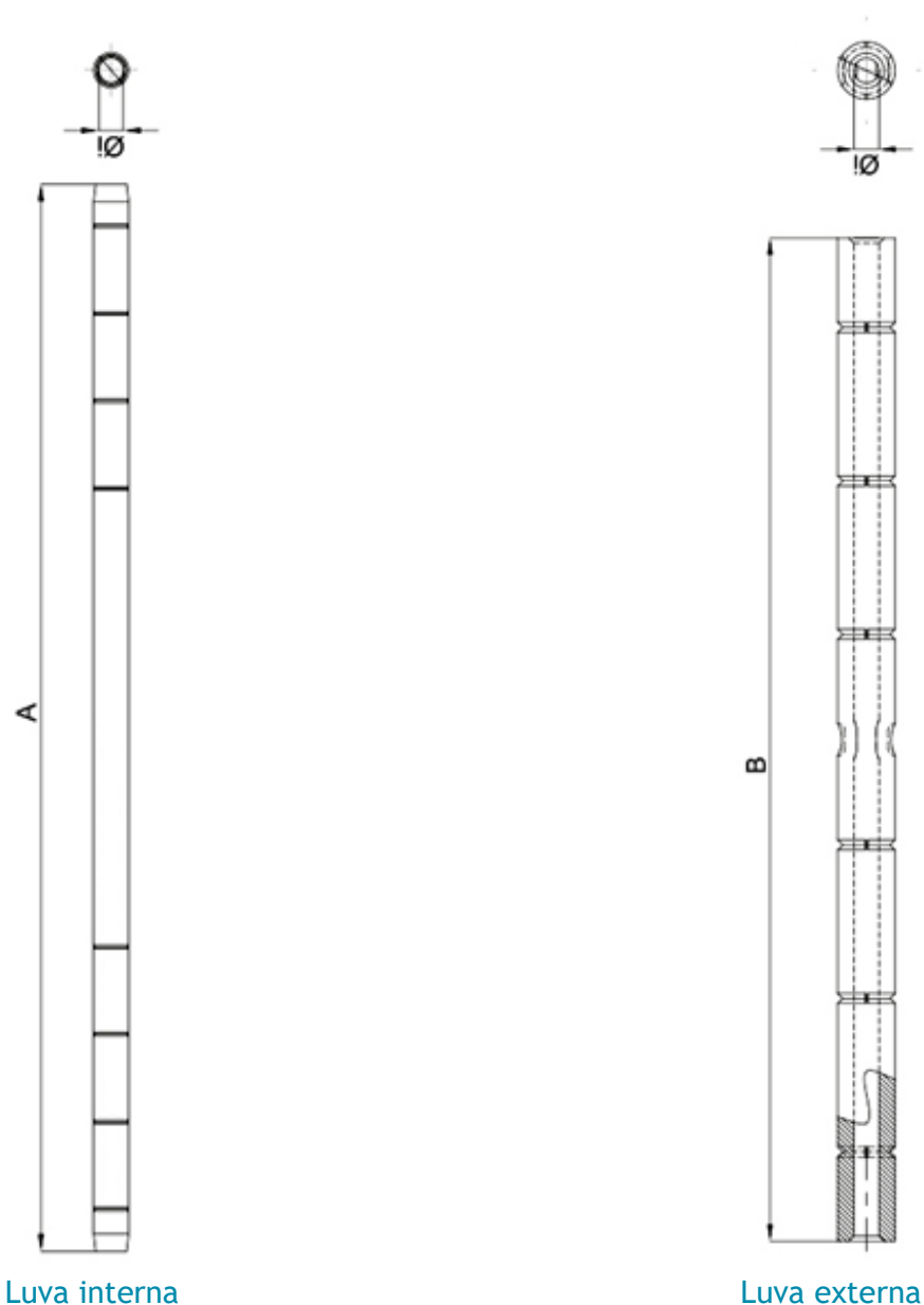
DESENHO 1 - Característica dimensional da luva de emenda de tração total para condutores alumínio CAA/ACSR e T-CAA/T-ACSR
