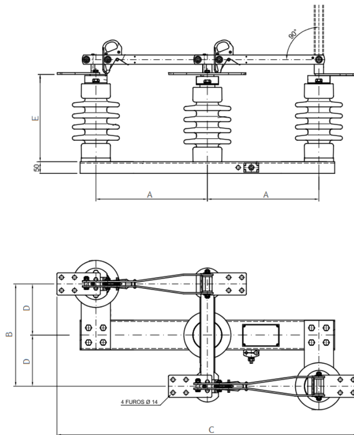
DESENHO 1 - Características dimensionais da chave seccionadora tipo tandem de subestação
