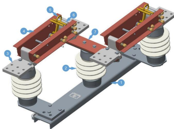
Figura 1 - Chaves seccionadoras tipo tandem (TD) até 36,2 kV
