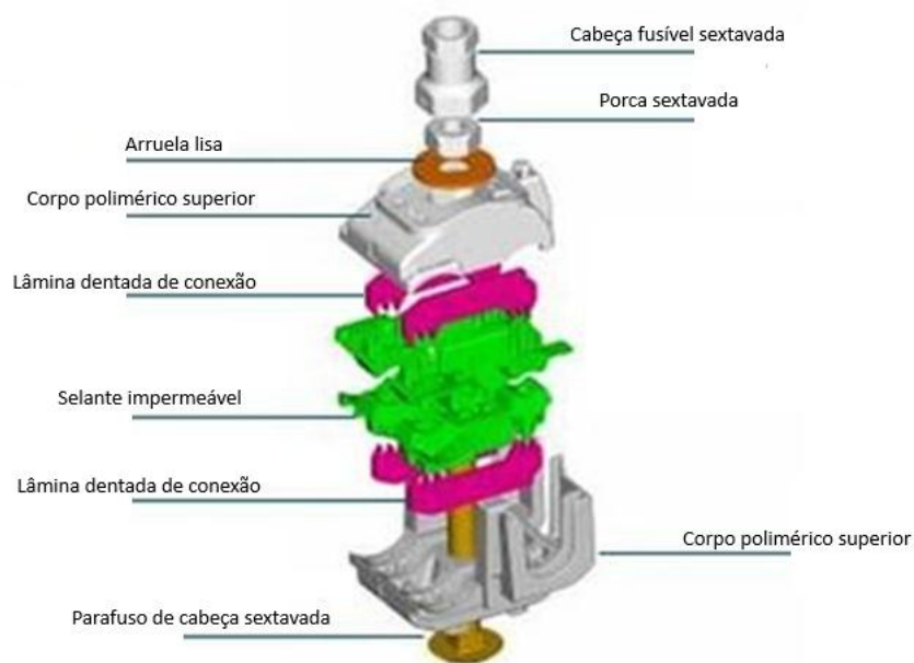
Figura 1 - Conector derivação perfurante de MT.
