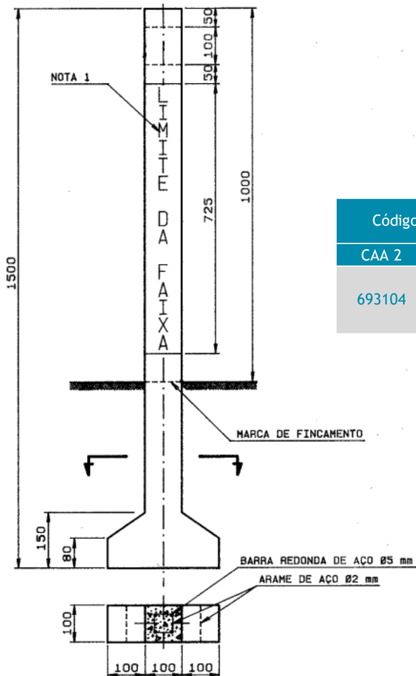
DESENHO 1 - Característica dimensional do marco de sinalização vertical para linhas de alta tensão de 145 kV
