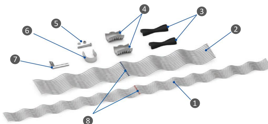
Figura 1 - Grampo de suspensão armado
