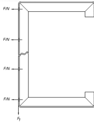
Figura 1 - Detalhe para execução do ensaio
