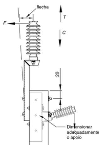
Figura 1 - Detalhe para execução do ensaio
