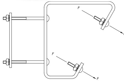
Figura 1 - Detalhe para execução do ensaio
