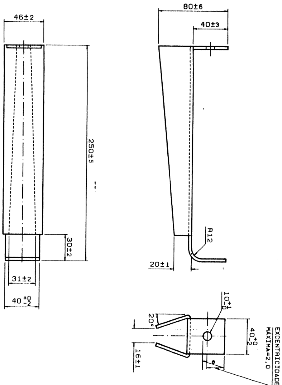
DESENHO 1 - Característica dimensional do suporte tipo bandeja para cabos isolados até 36,2 kV
