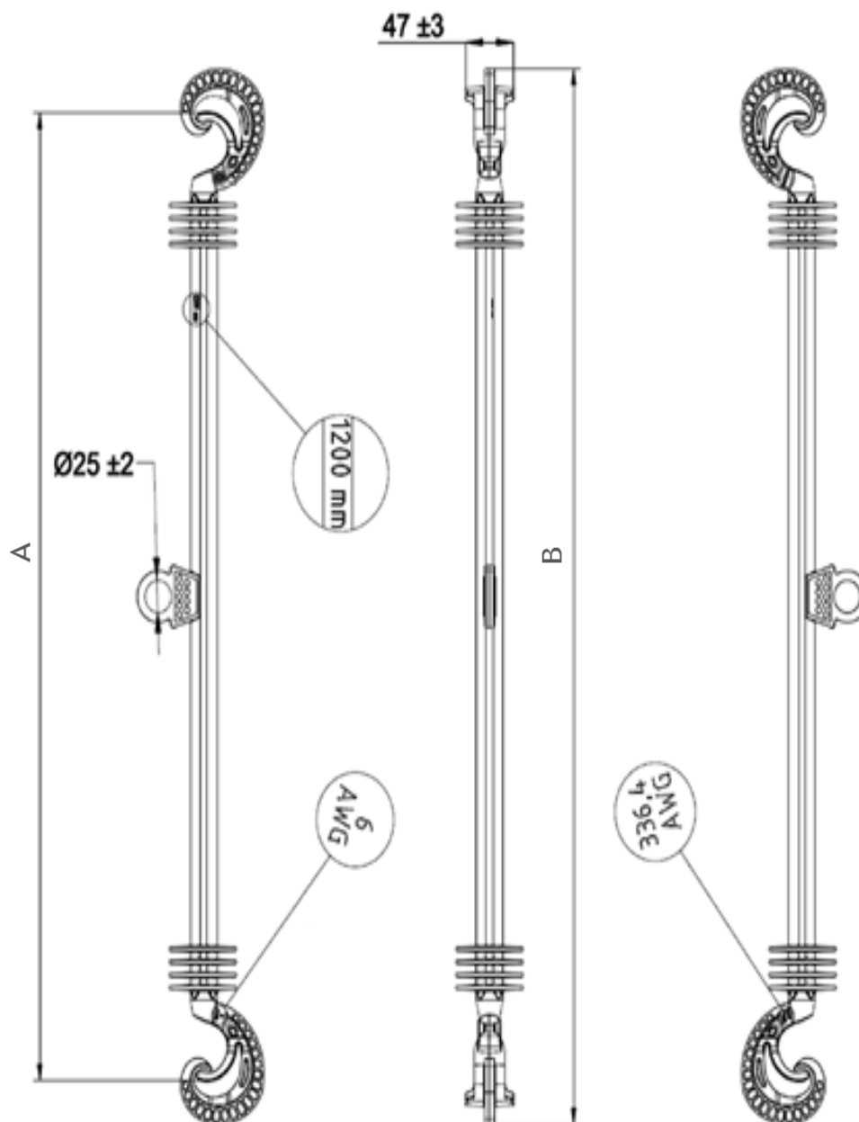
DESENHO 1 - Características dimensional do espaçador horizontal de média tensão convencional
