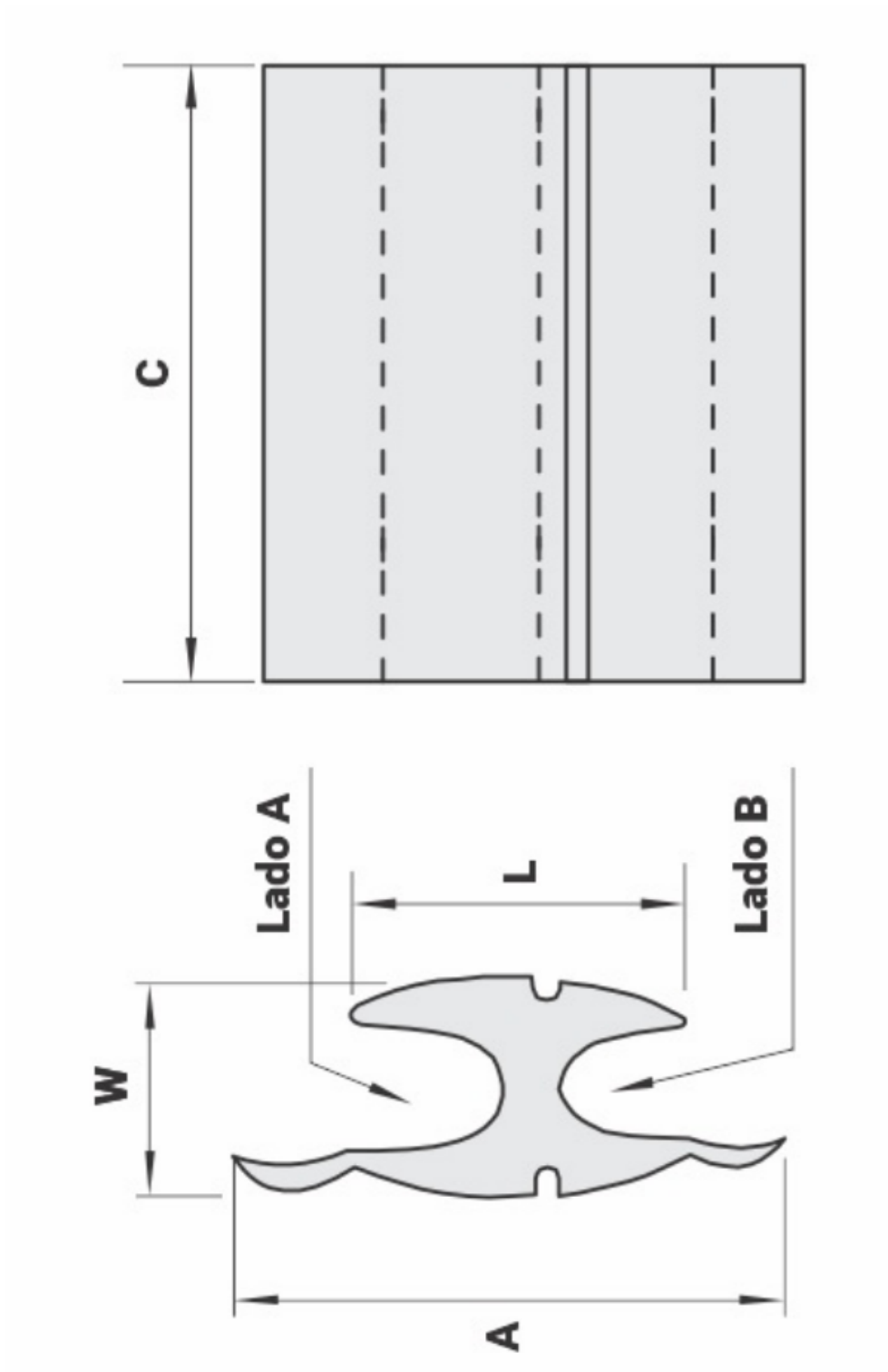
DESENHO 1 - Característica dimensional do conector de derivação à compressão do tipo H
