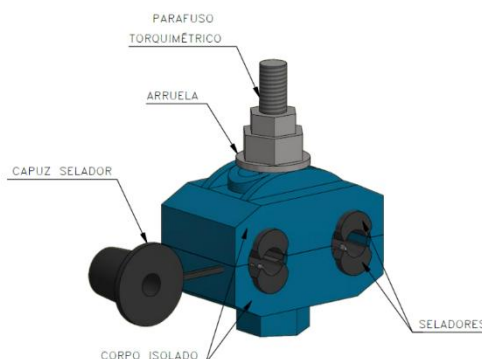
Figura 1 - Conector derivação perfurante para rede secundária isolada.
