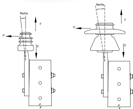
Figura 1 - Detalhe para execução do ensaio
