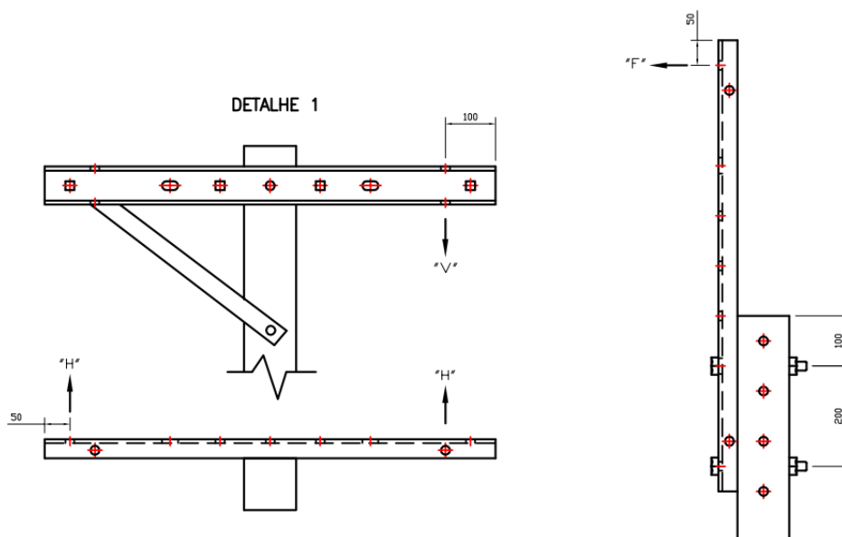
Figura 1 - Detalhe para execução do ensaio
