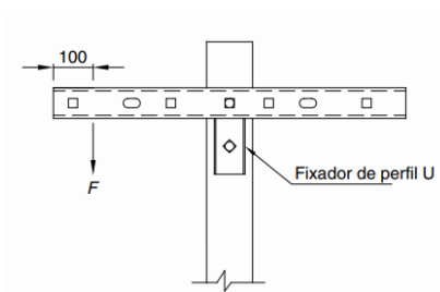
Figura 1 - Detalhe para execução do ensaio
