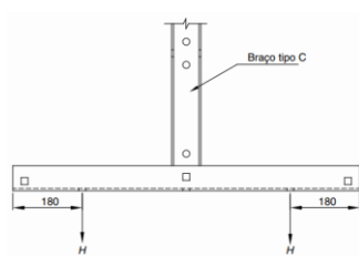
Figura 1 - Detalhe para execução do ensaio
