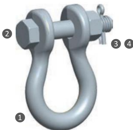
Figura 1 - Manilhas metálicas para redes de distribuição até 145 kV
