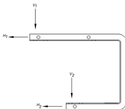
Figura 1 - Detalhe para execução do ensaio
