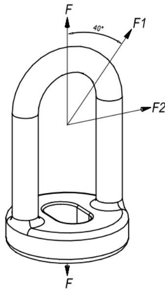
Figura 1 - Detalhe para execução do ensaio
