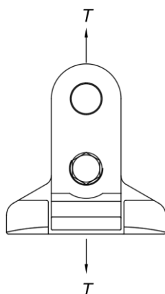
Figura 1 - Detalhe para execução do ensaio
