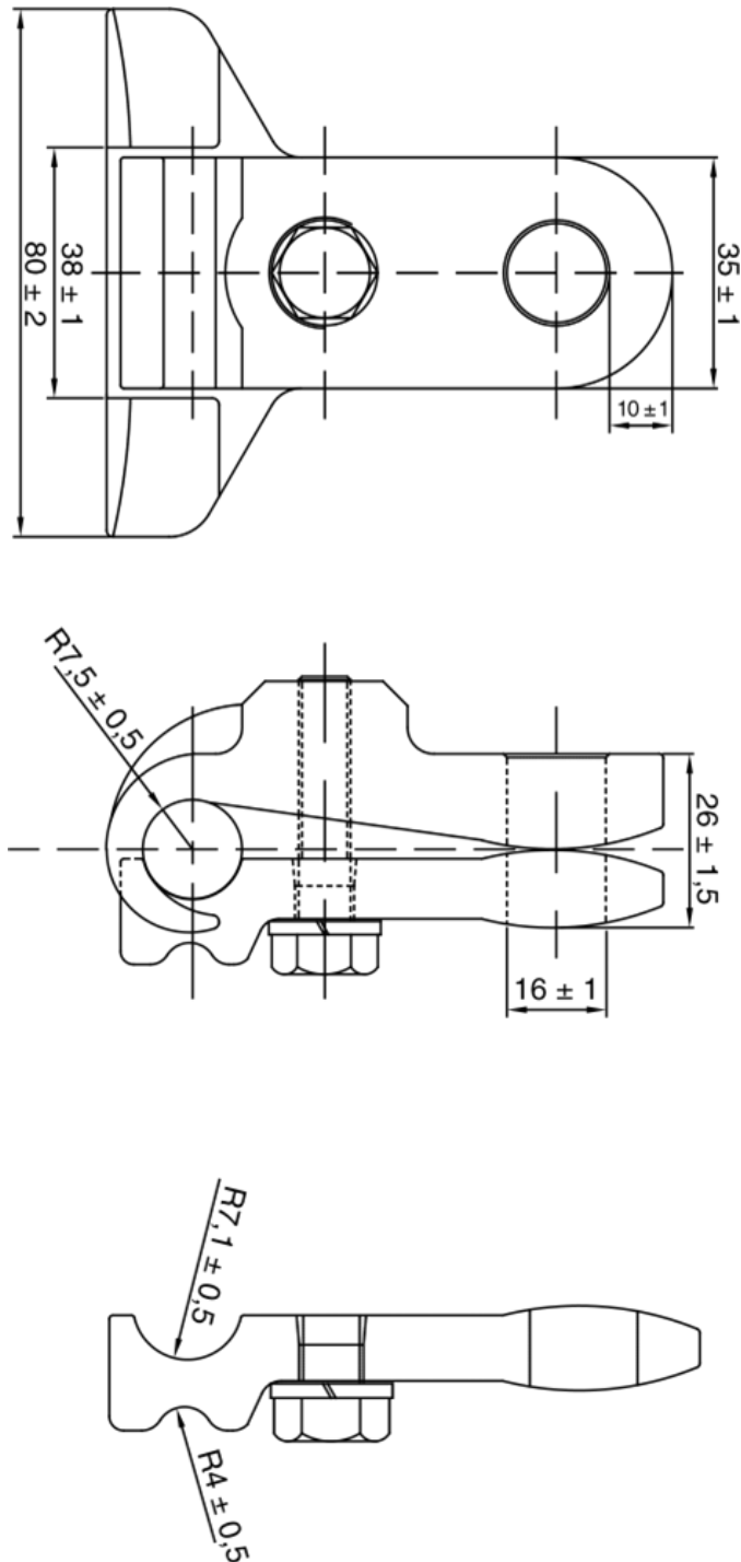
DESENHO 1 - Características dimensionais do grampo de suspensão
