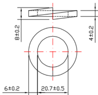
Arruela de Pressão M-20
