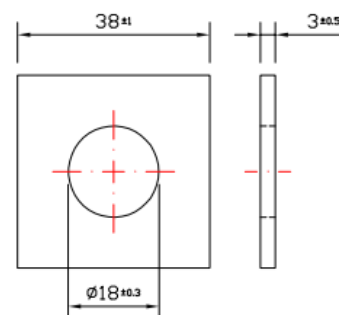
Arruela Quadrada 38x18x3
