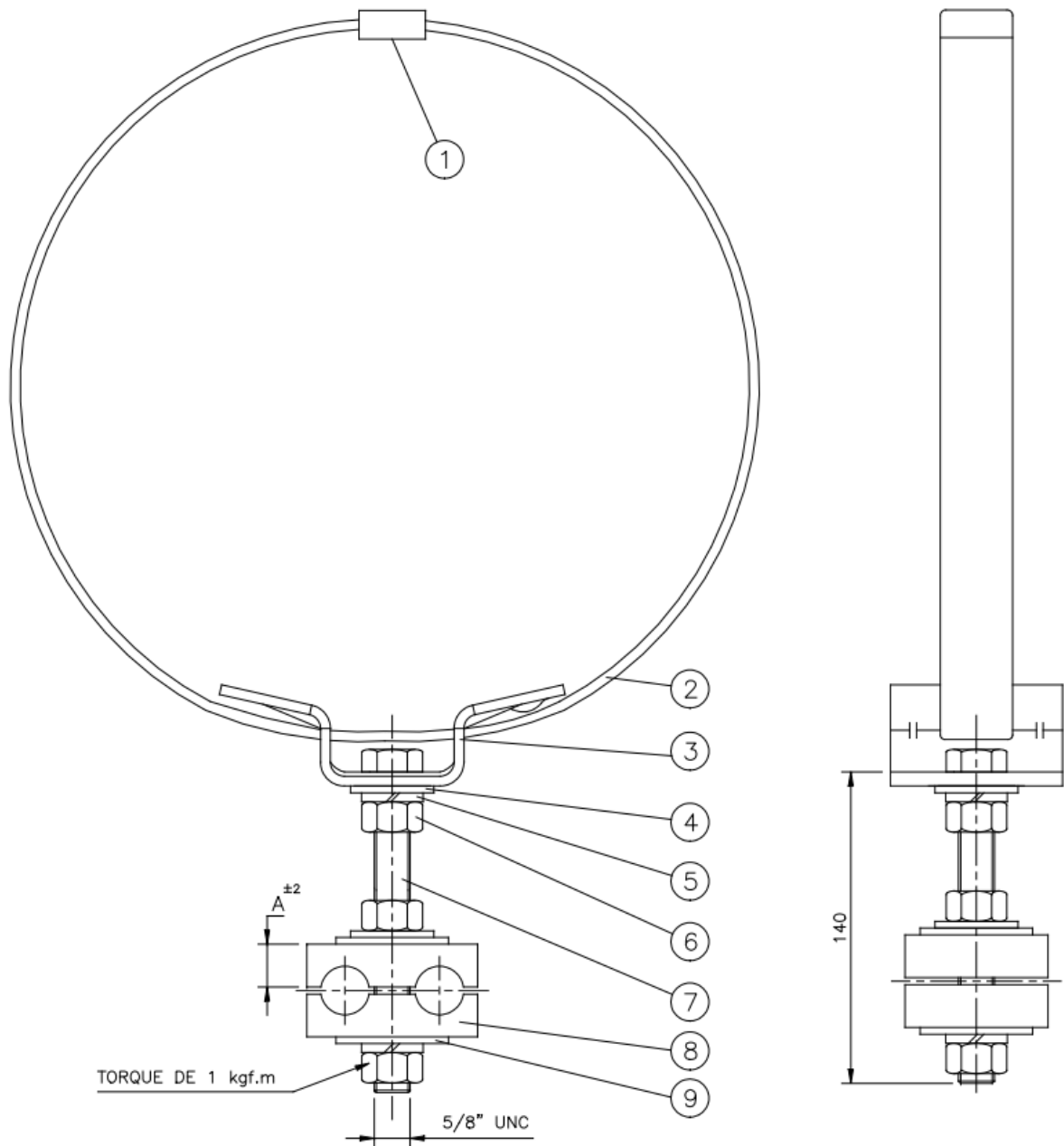
DESENHO 1 - Características dimensionais do conjunto grampo guia de descida para postes circulares
