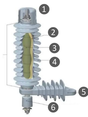
Figura 1 - Para-raios de distribuição
