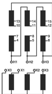
Figura 3 - Transformador trifásico - Diagrama de ligação (Dyn1)
