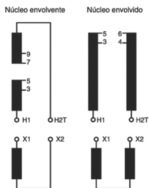
Figura 2 - Transformador monofásico - Diagrama de ligação
