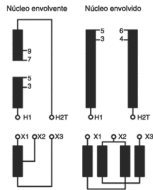
Figura 2 - Transformador monofásico - Diagrama de ligação
